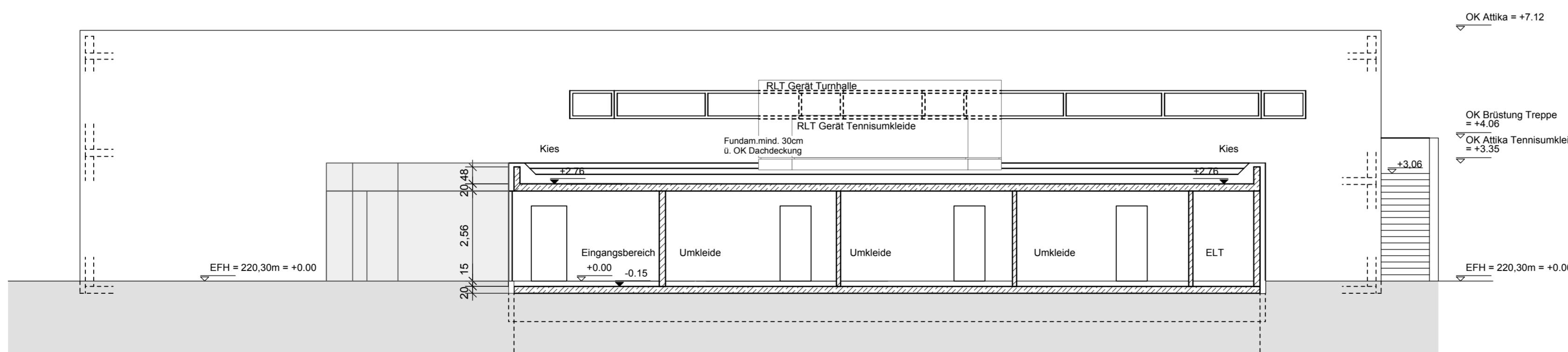
Schnitt B-B
