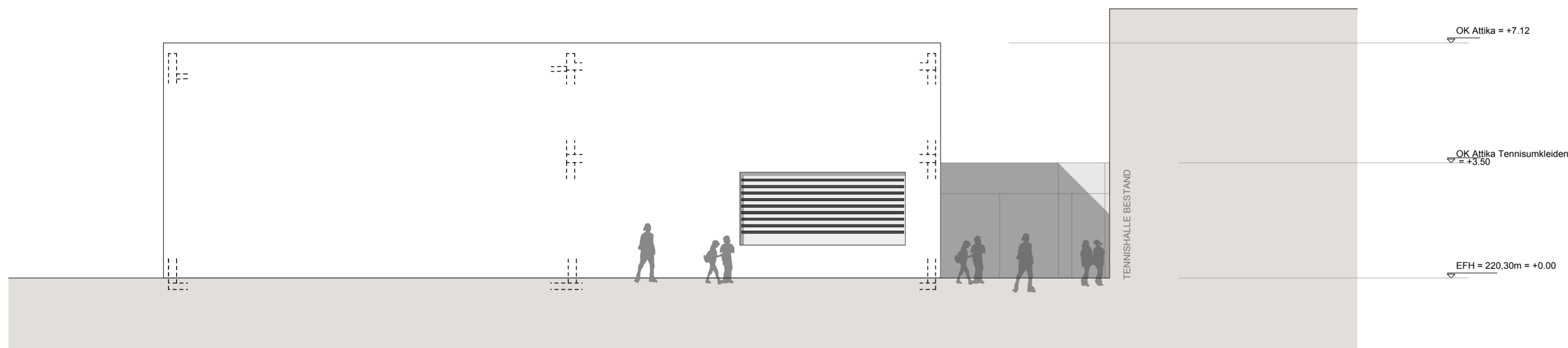
Ansicht Ost
