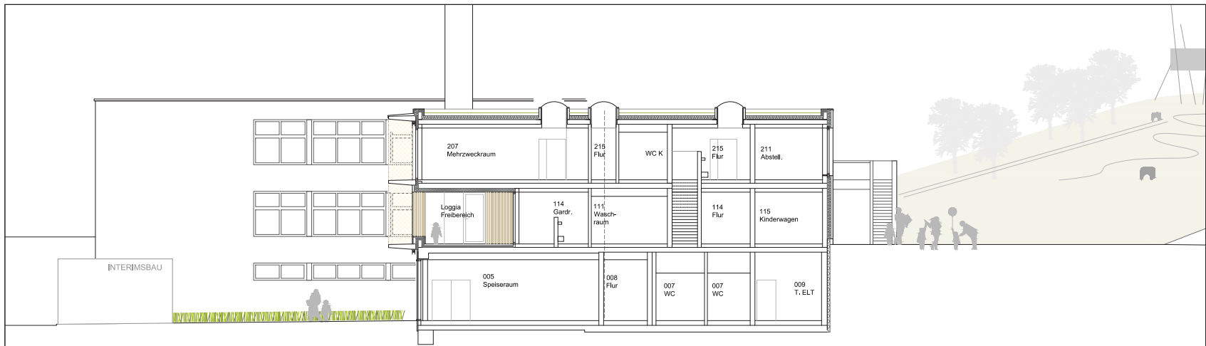
SCHNITT A-A
