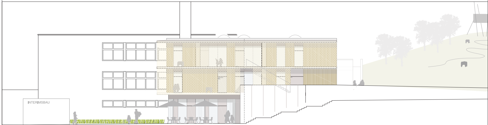
ANSICHT NORD-OST
