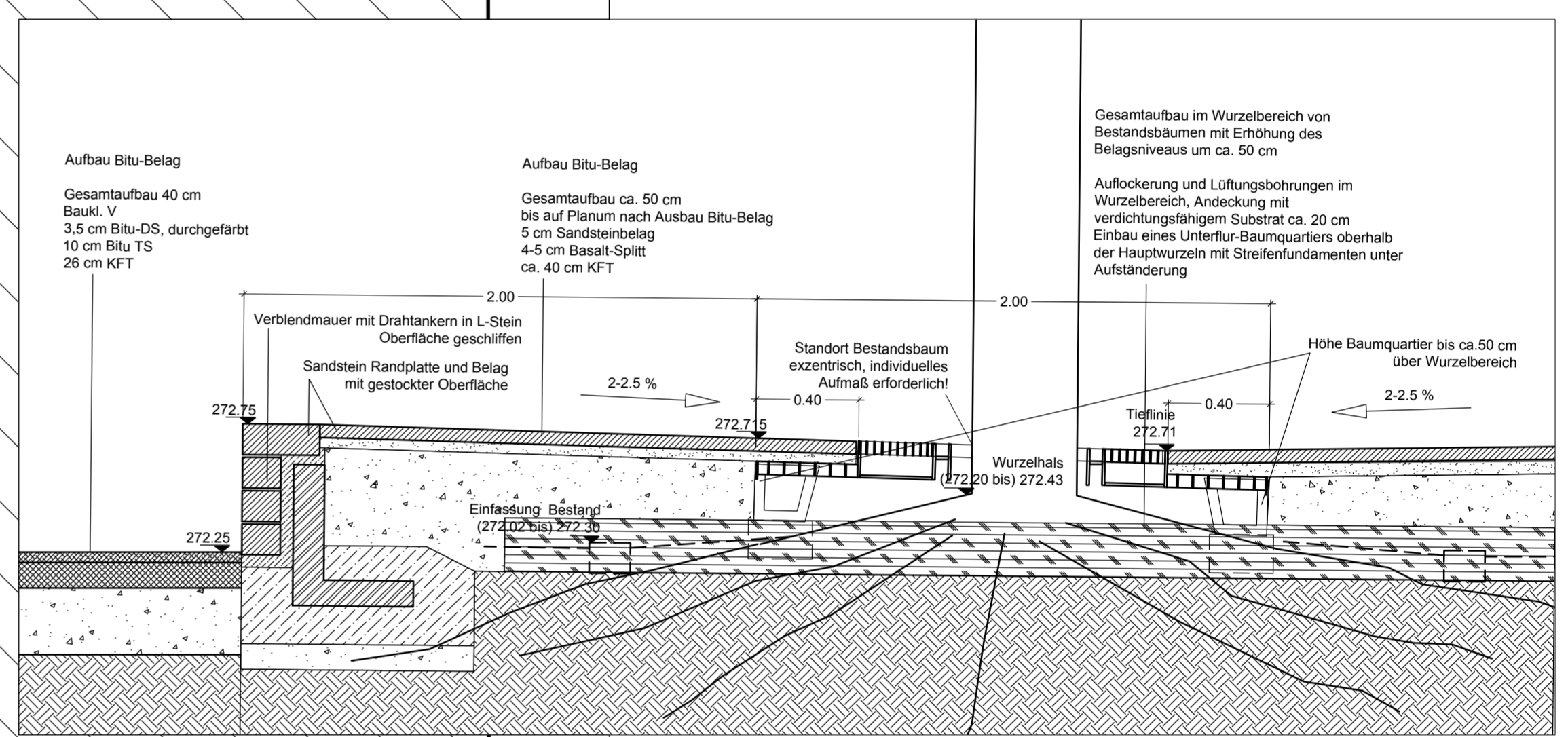
Schnitt 1-1 | Plattform mit Bestandslinden in Baumquartieren
