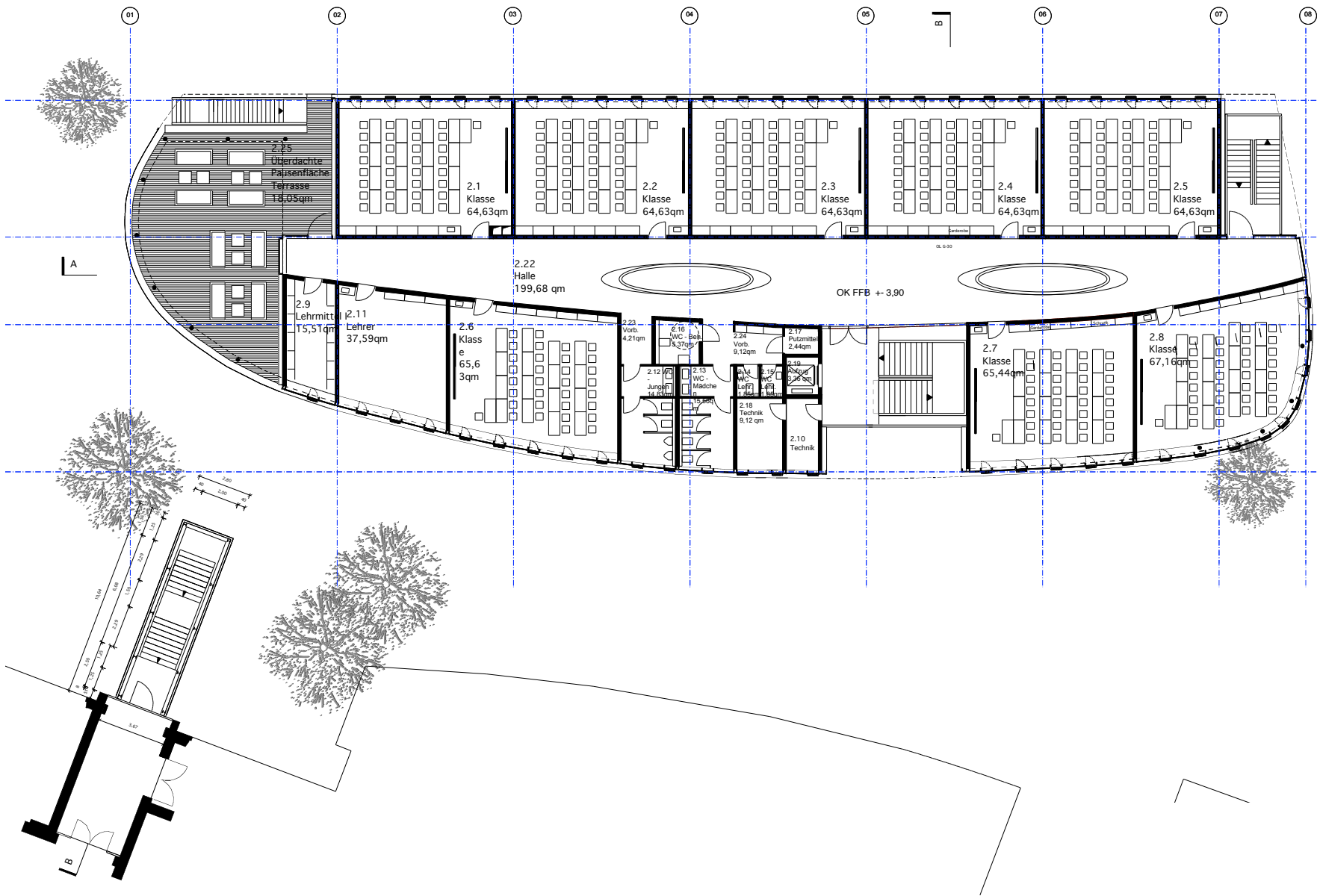
Grundriss OG
