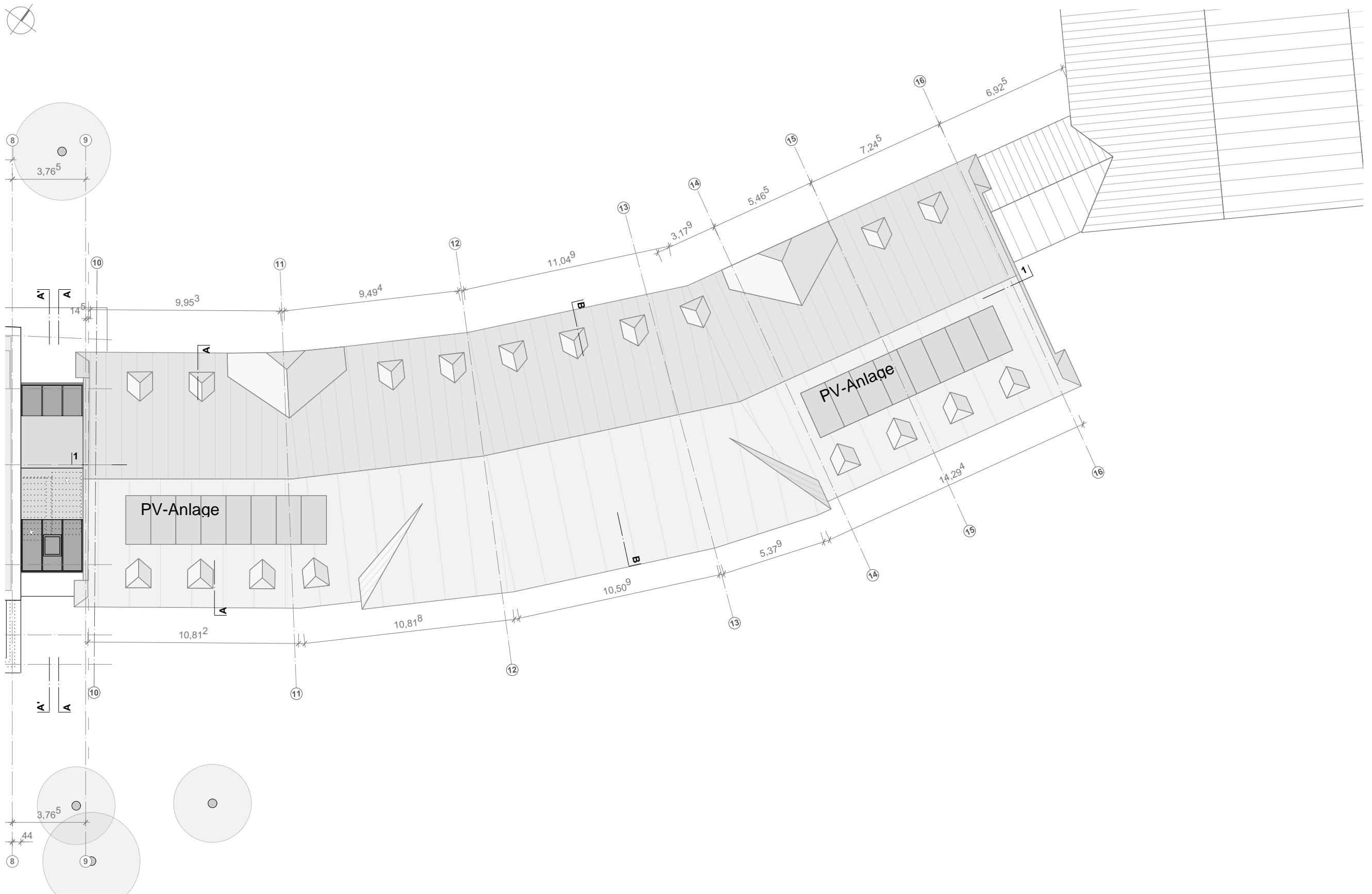
Grundschule Kaltental Sanierung Bestand I 21.08.2023 | o.M. | Grundriss Dachaufsicht
