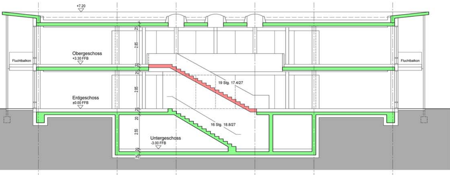
Schnitt A-A
