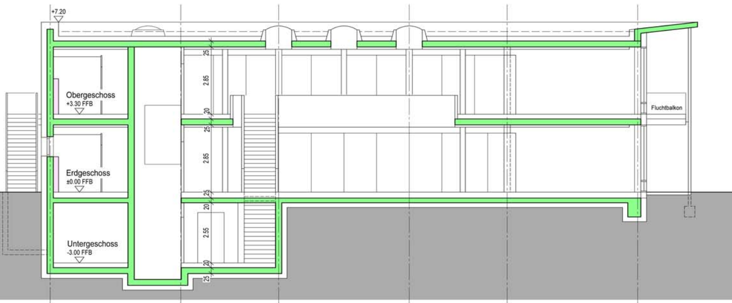
Schnitt A-A
