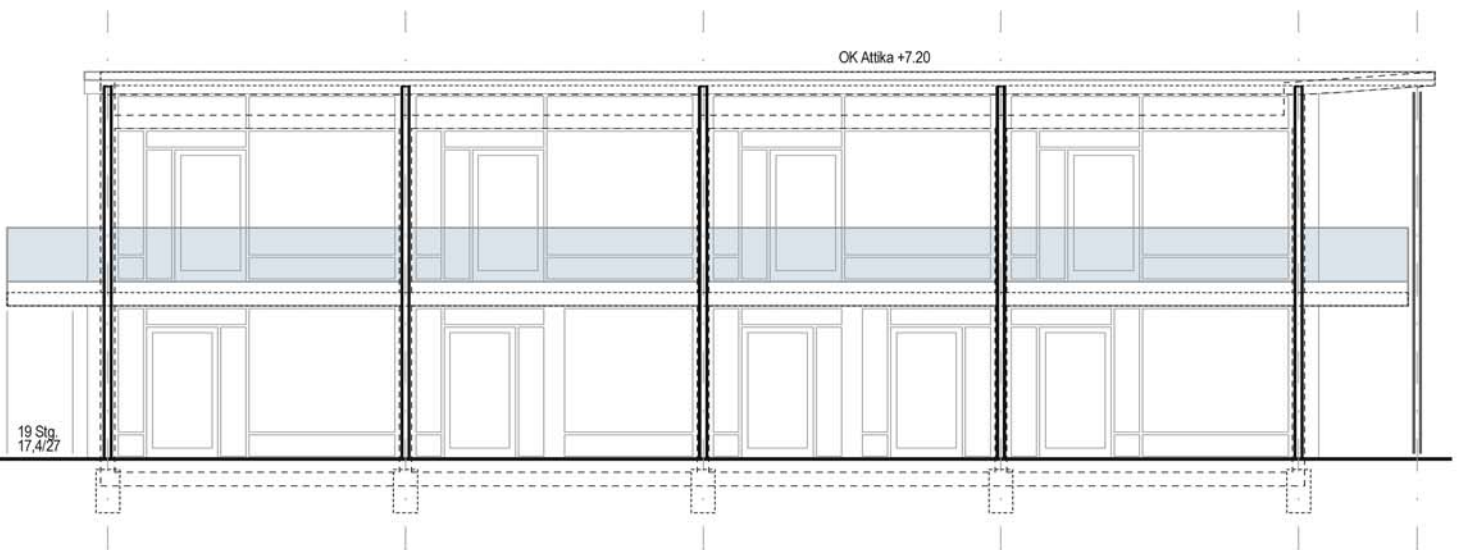
Ansicht Garten
