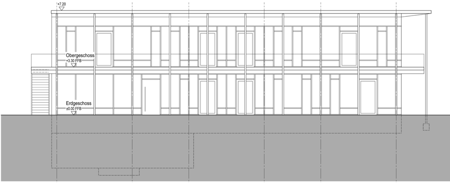
Ansicht Eingang
