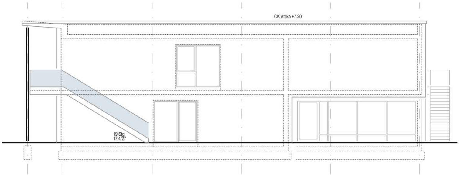
Ansicht Eingang
