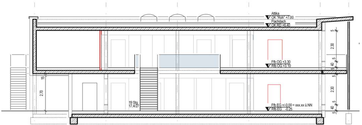
Schnitt A-A
