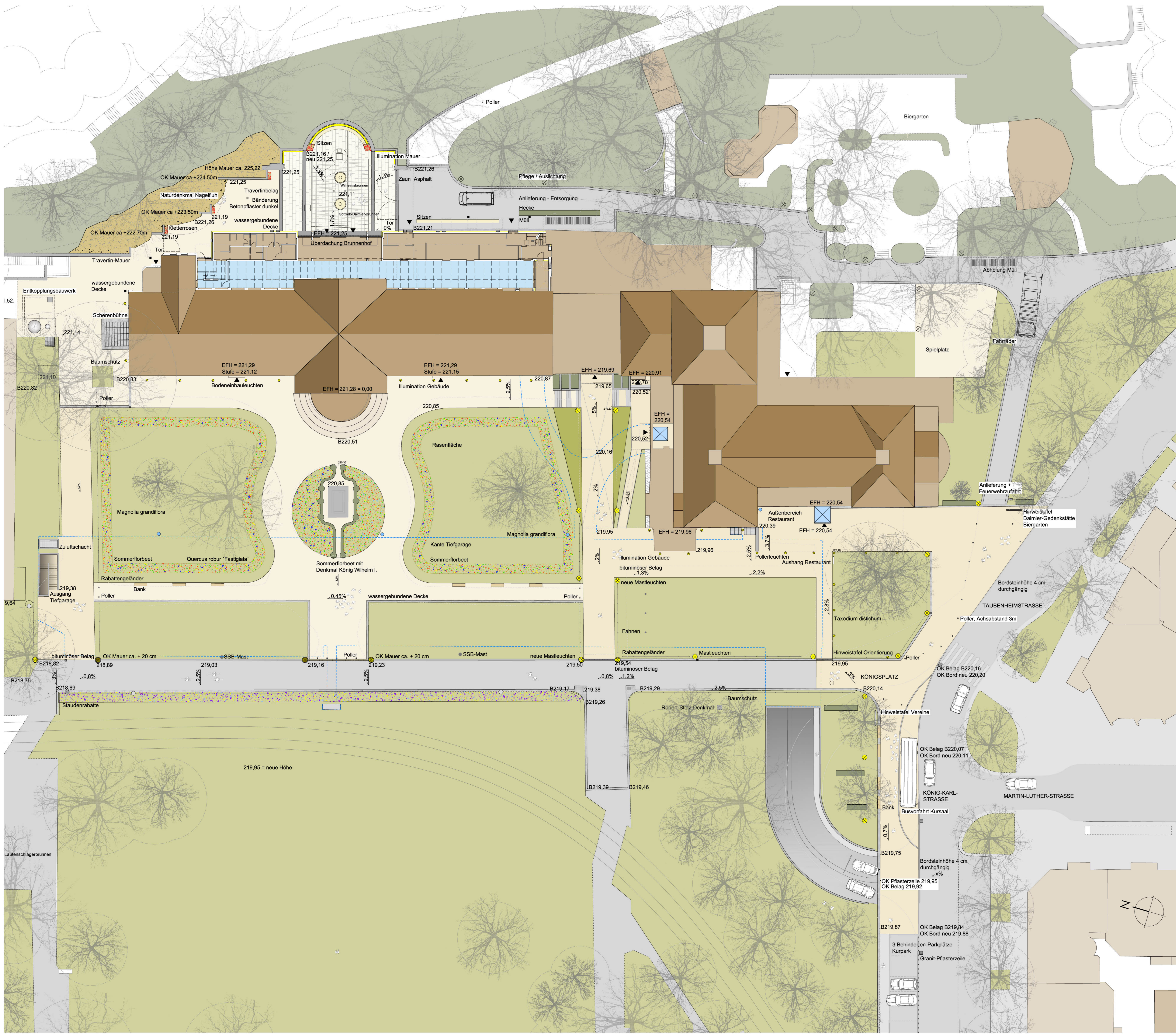
Lageplan M 1:200
