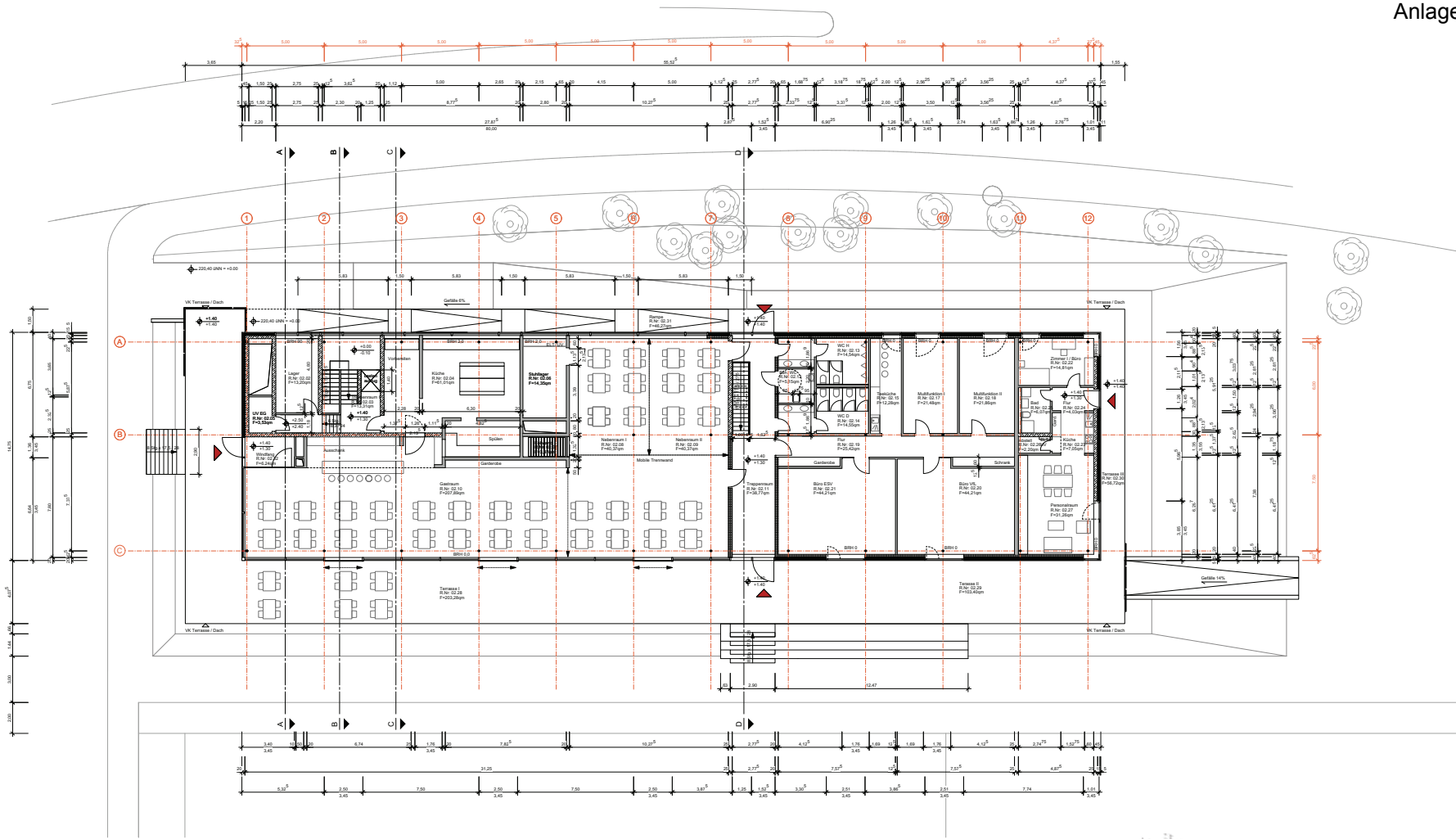
Grundriss EG
