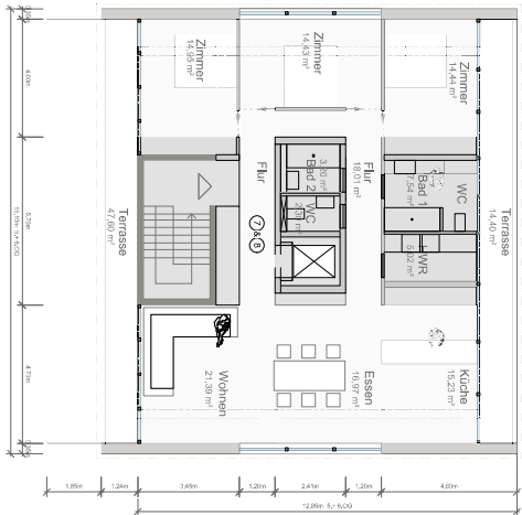
Grundriss OG 4.5 M 1:100
