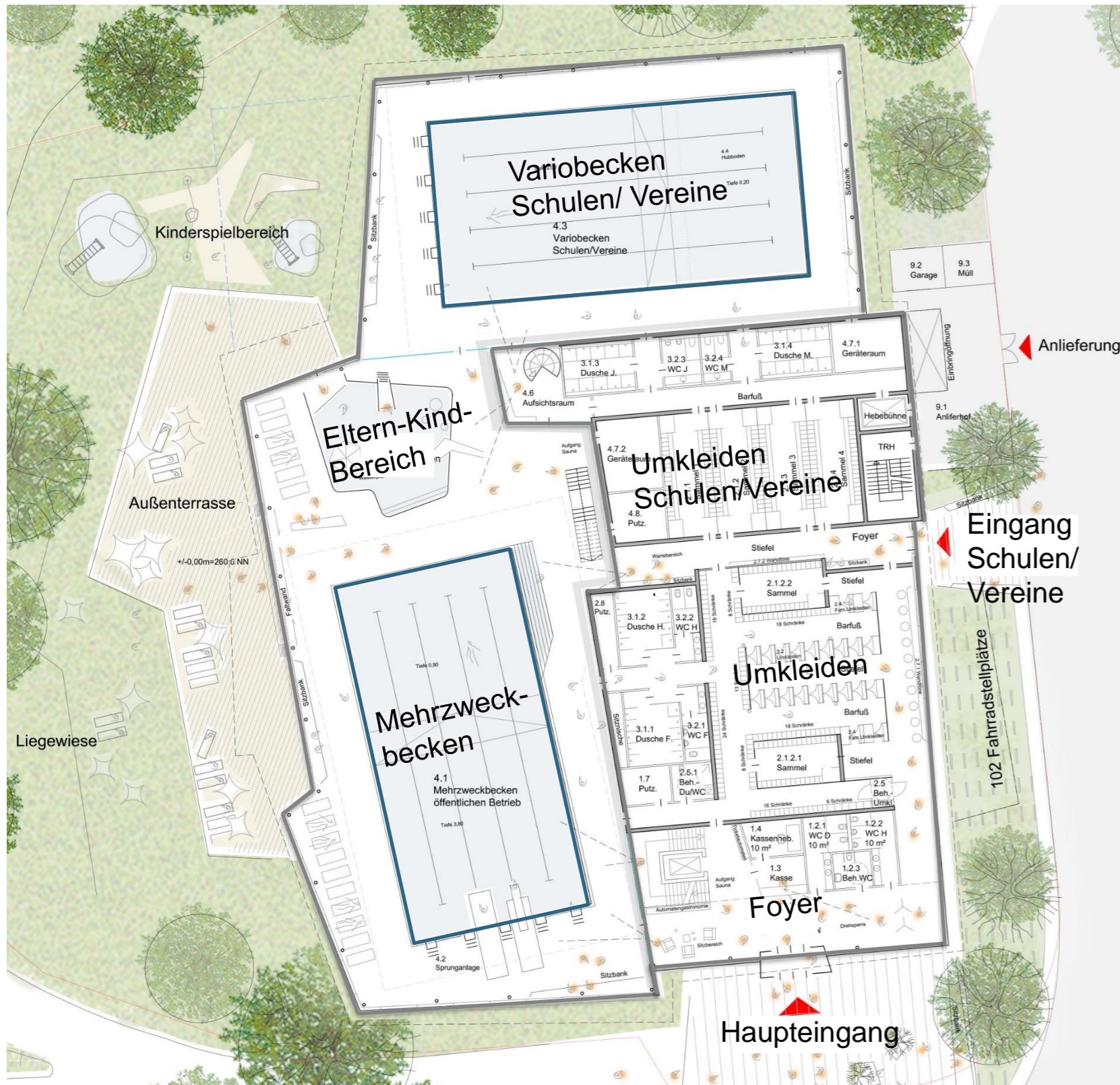
Grundriss Erdgeschoss
