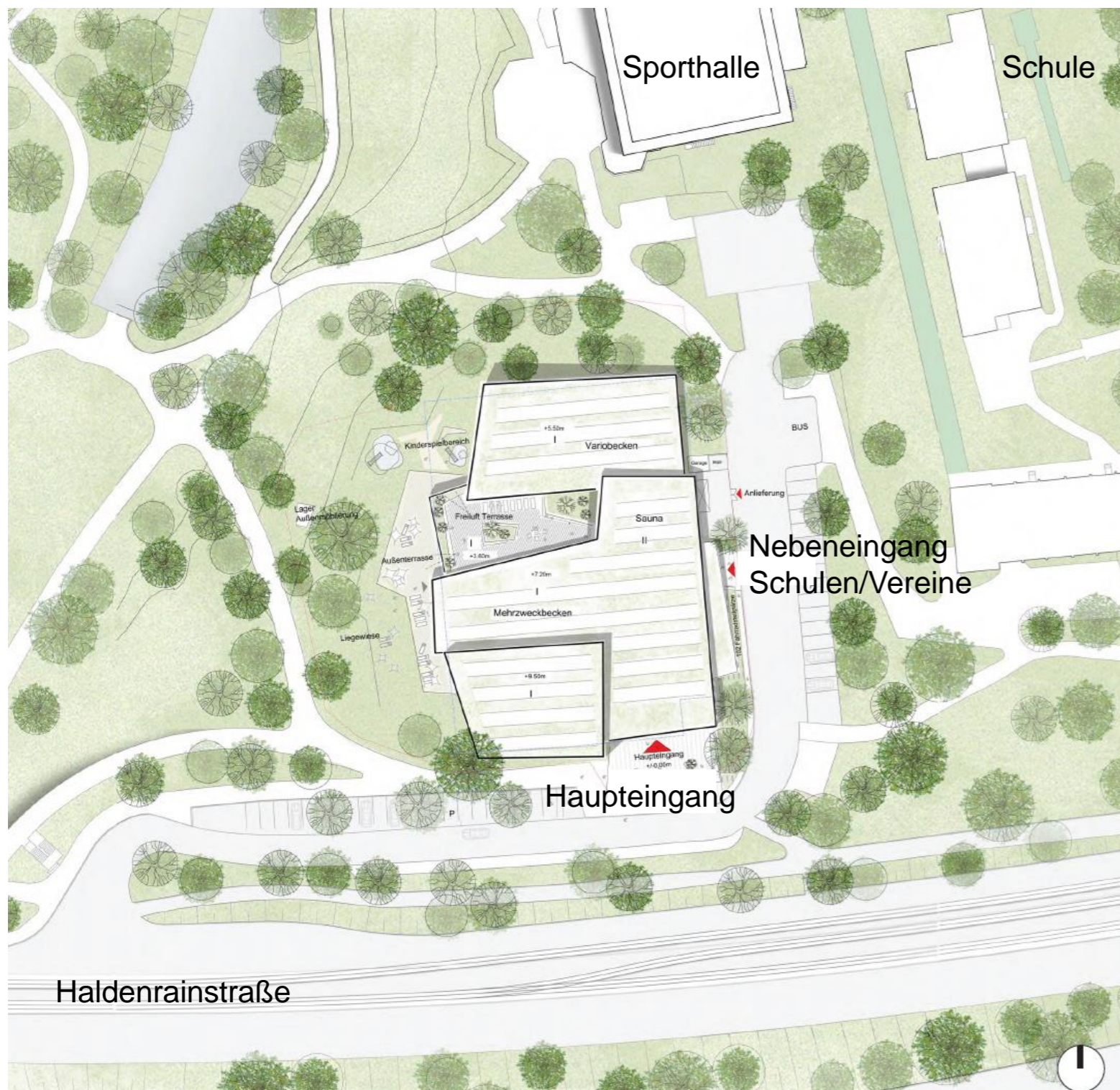
Lageplan
