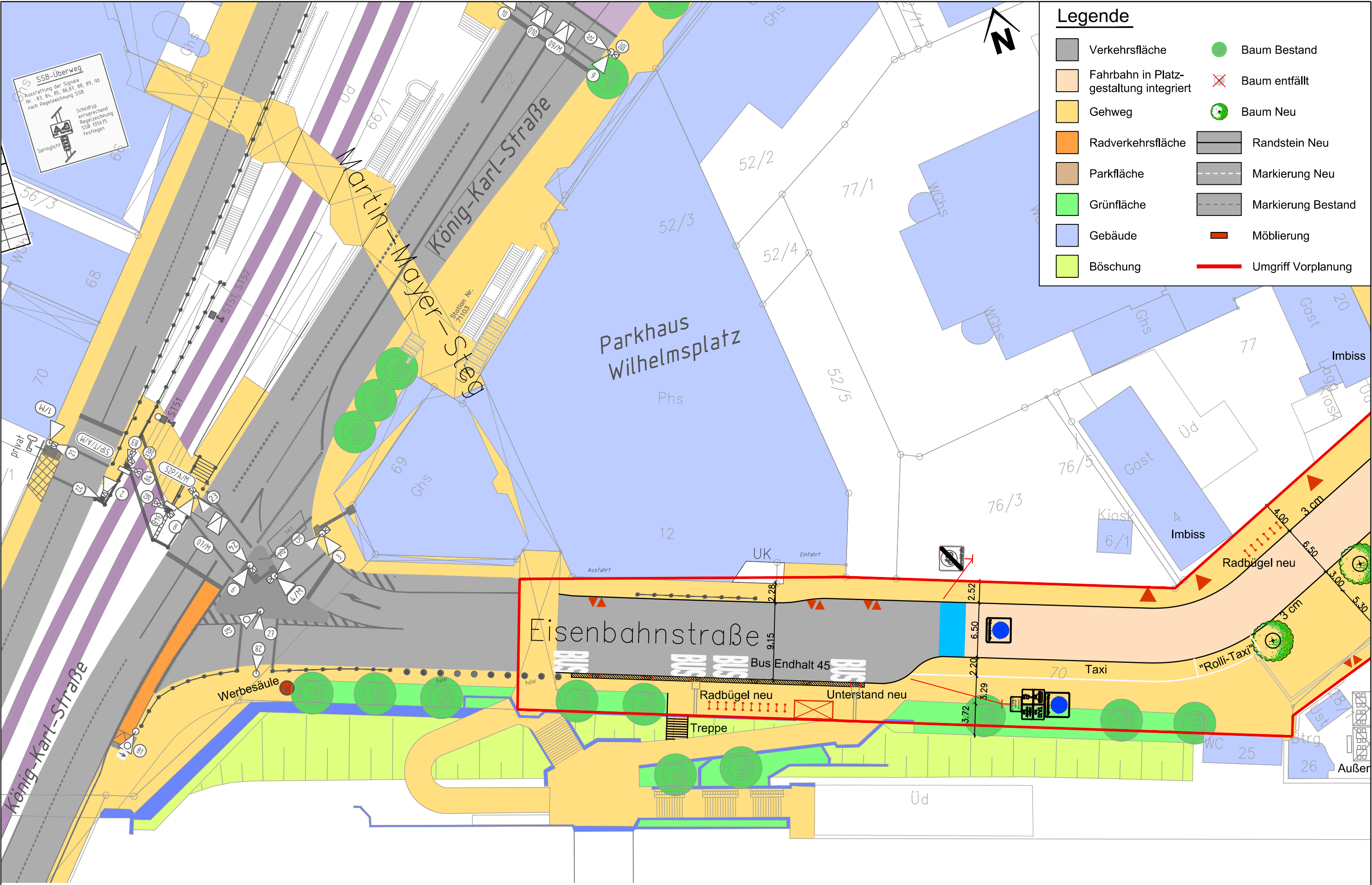
Stuttgart-Bad Cannstatt Vorplanung Umgestaltung Bahnhofsvorplatz / Blatt 1
