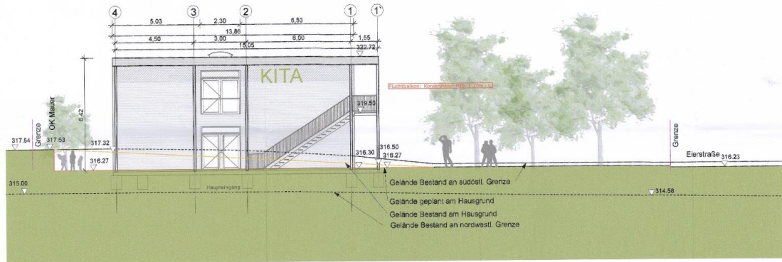
Ansicht Südost
