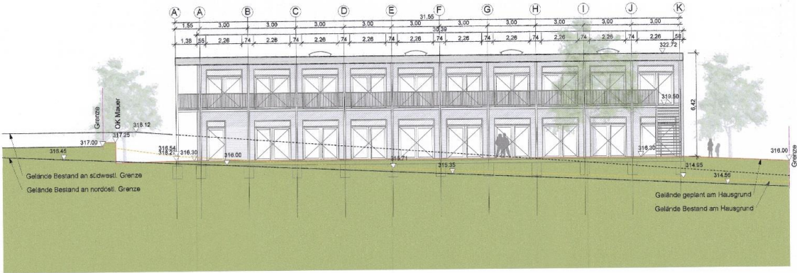
Ansicht Nordost
