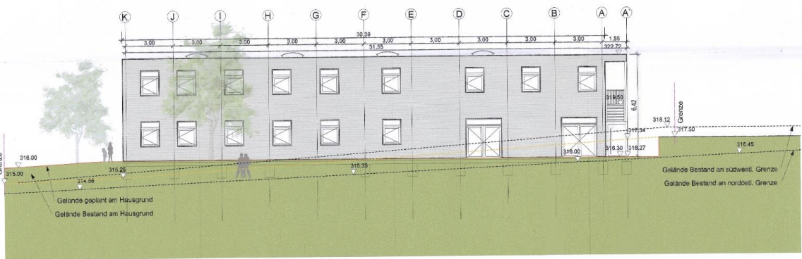
Ansicht Südwest
