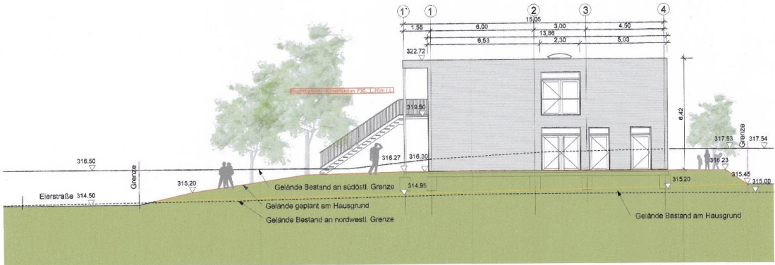
Ansicht Nordwest
