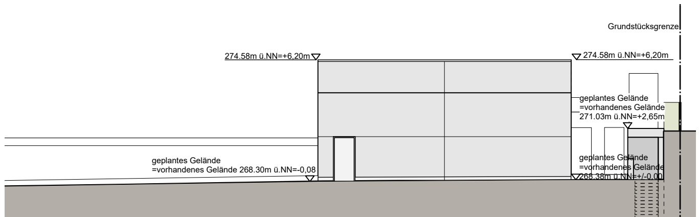
Ansicht West
