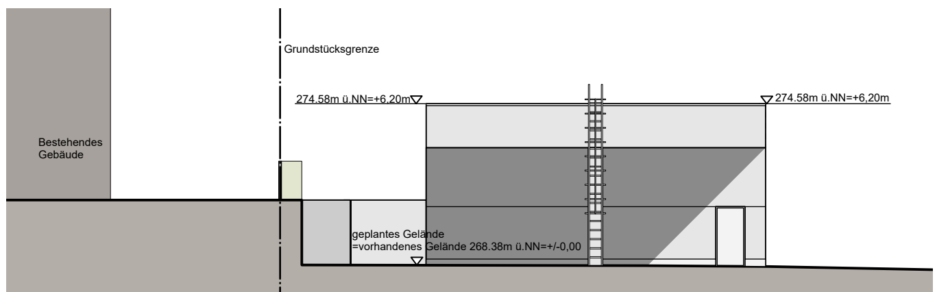
Ansicht Ost
