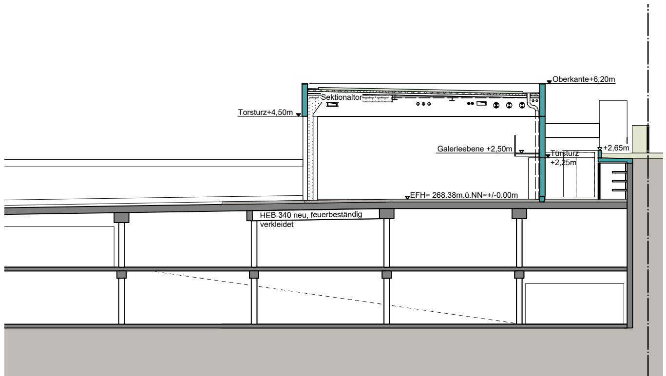
Querschnitt
