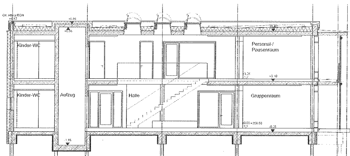
Schnitt
