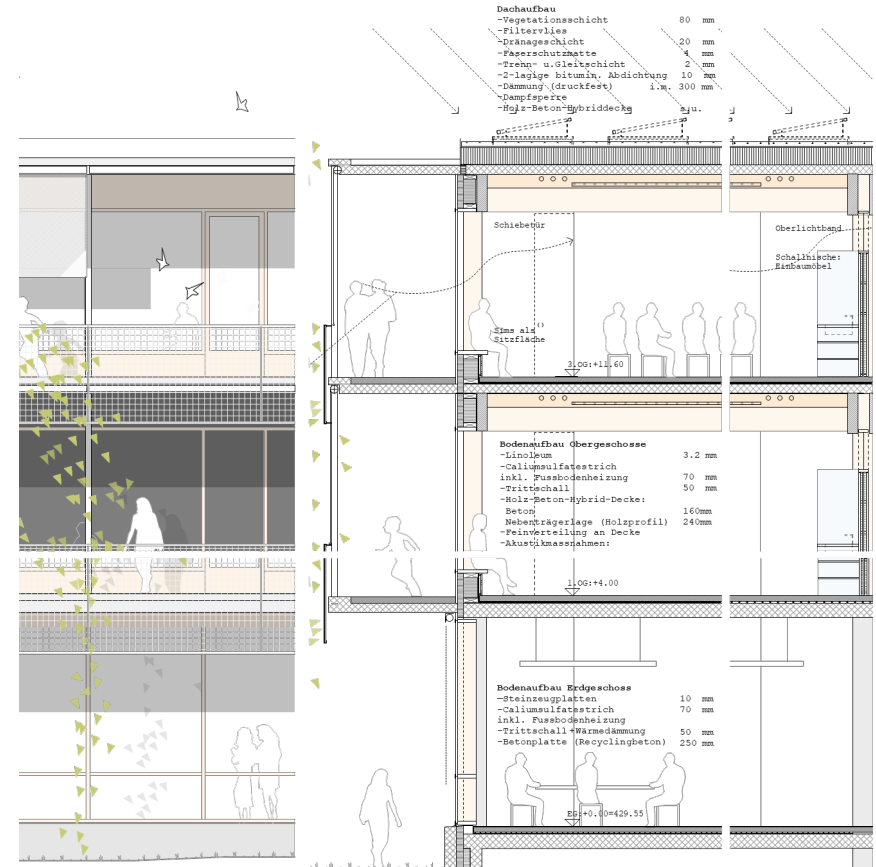
Fassade | Fassadenschnitt
