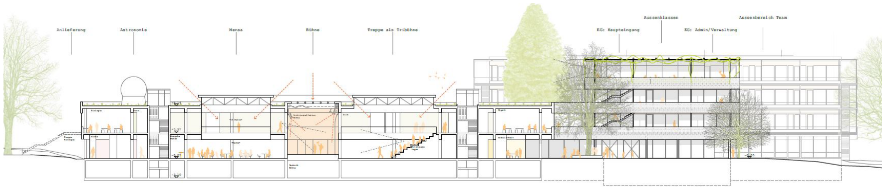
Längsschnitt Bestand | Ansicht Neubau mit Haupteingang Schule
