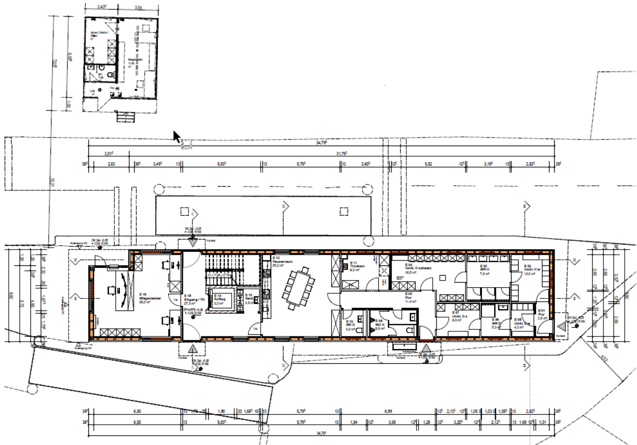
Grundriss EG
