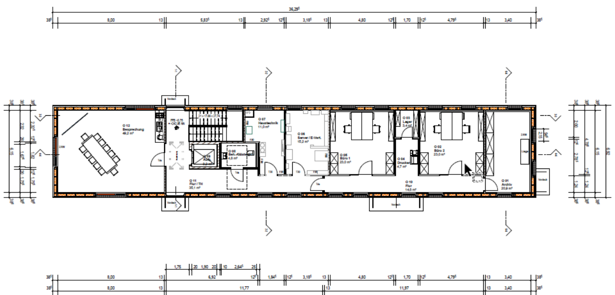
Grundriss OG
