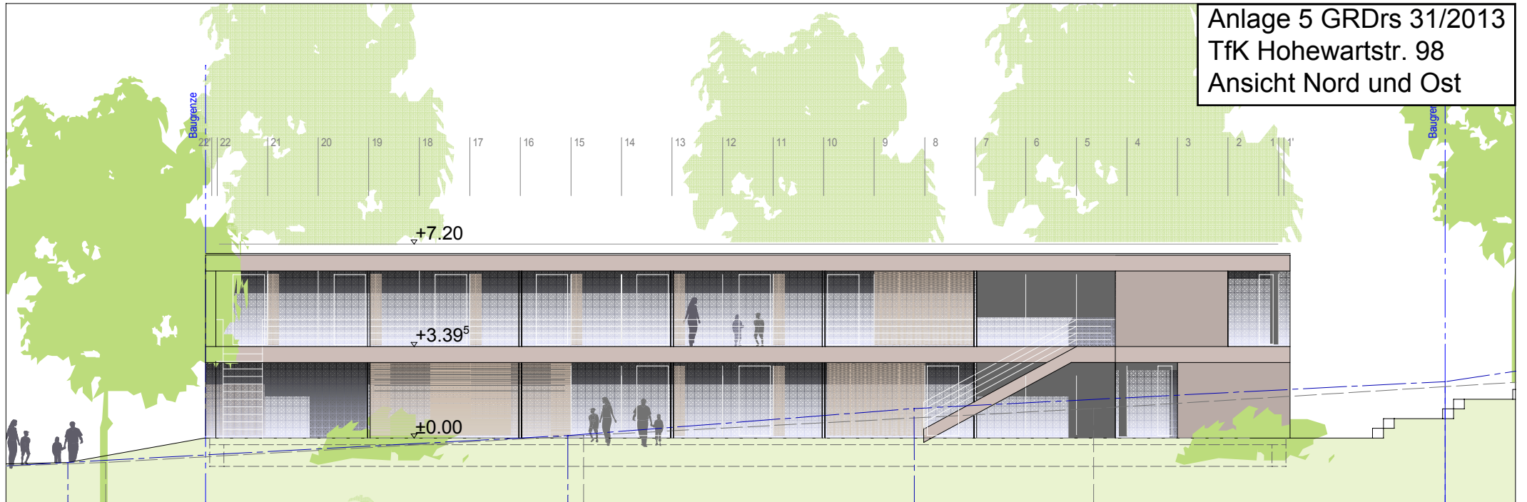
Ansicht Nord
