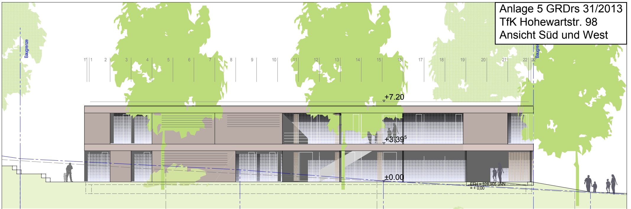
Ansicht Süd
