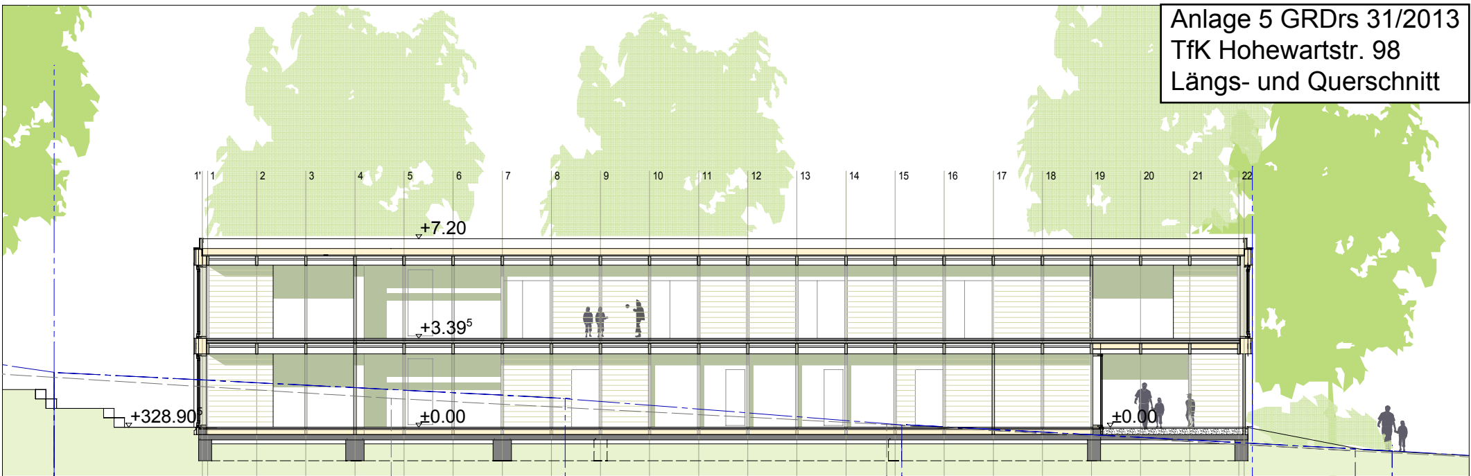
Schnitt L 1
