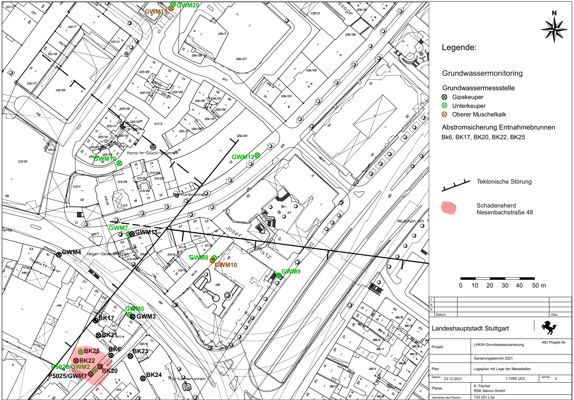
Abbildung: Grundwassermonitoring im Abstrom und Abstromsicherung während Sanierung, Nesenbachstraße 48
