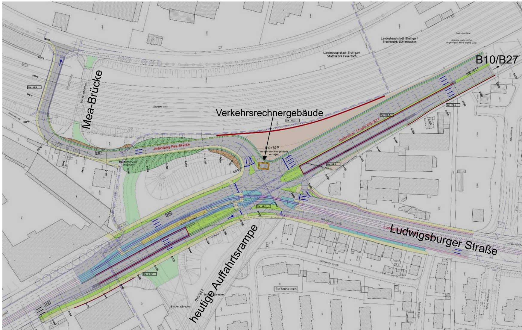
Lageplan der Vorzugsvariante (Machbarkeitsstudie 2008)
