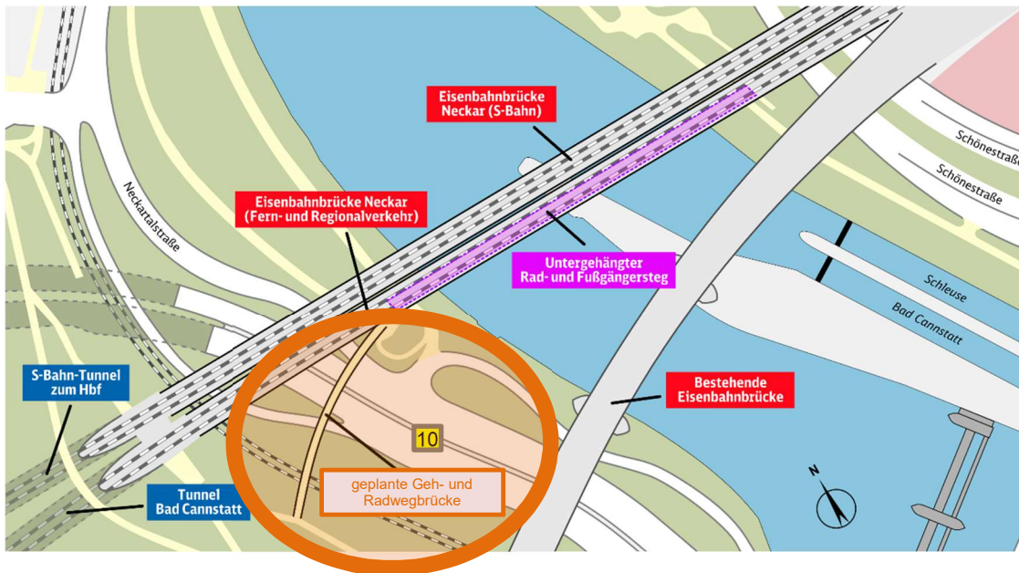
Abb. 1: Lageplan der geplanten Geh- und Radwegbrücke über die B 10 Neckartalstraße
