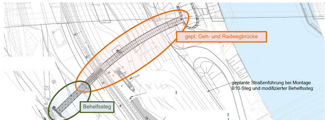
Abb. 2: Lageplan der geplanten Geh- und Radwegbrücke über die B 10 Neckartalstraße mit Behelfssteg
