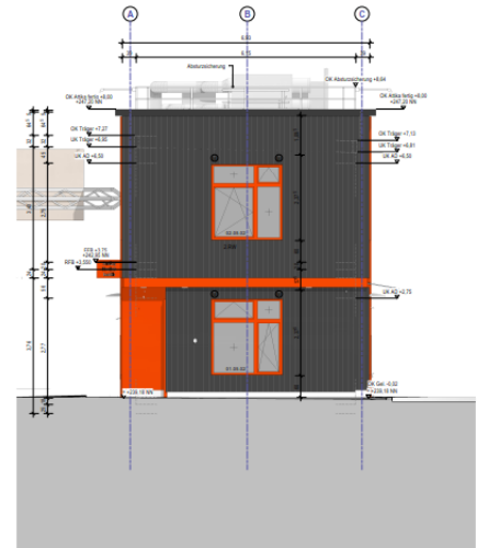
Ansicht Süd
