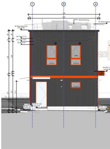
Ansicht Nord
