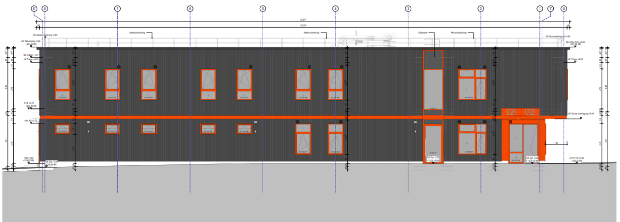
Ansicht West
