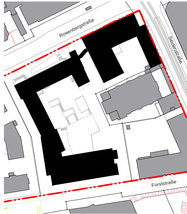
Lageplan Bestand rechtskräftige Baulinie nach Bebauungsplan
