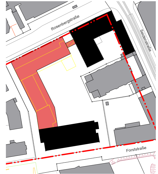
Neubau Gebäude Rosenbergstraße Empfehlung neue Baulinie gemäß Rahmenplan Talgrund West
