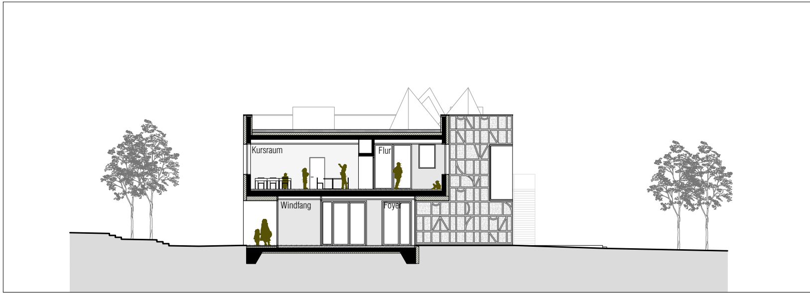
SCHNITT I-I'
