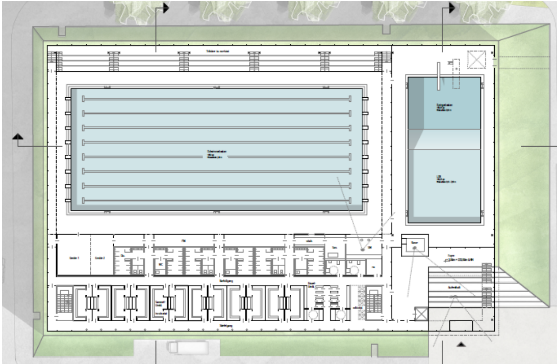
Grundriss EG mit Badeplatte
