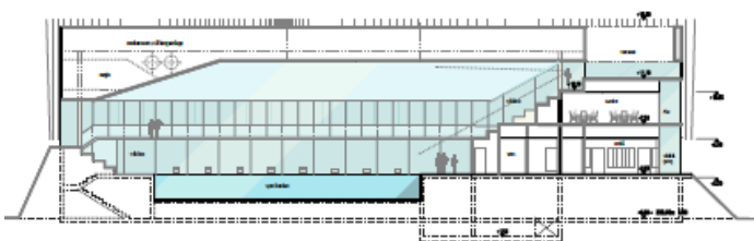
Schnitt C-C_M 1 : 200
