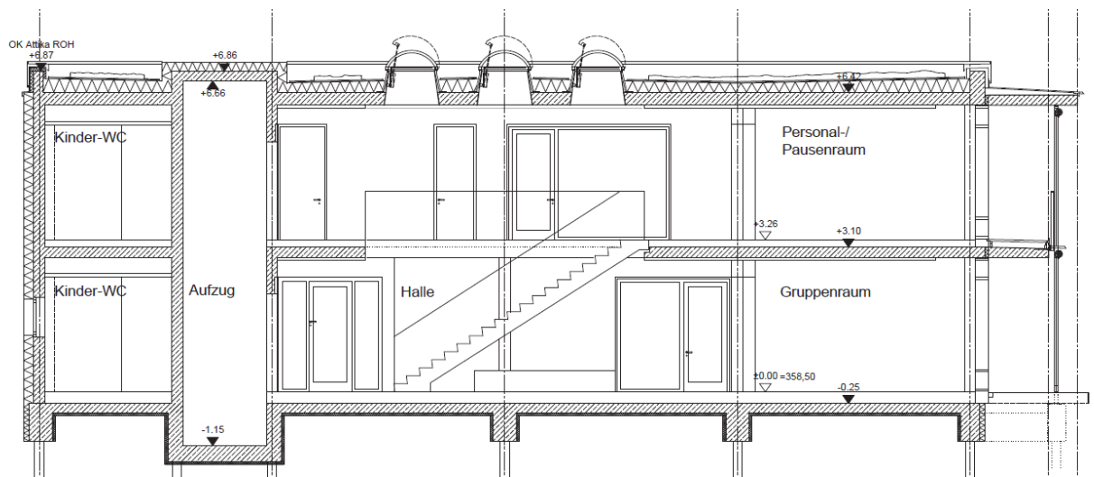
Schnitt
