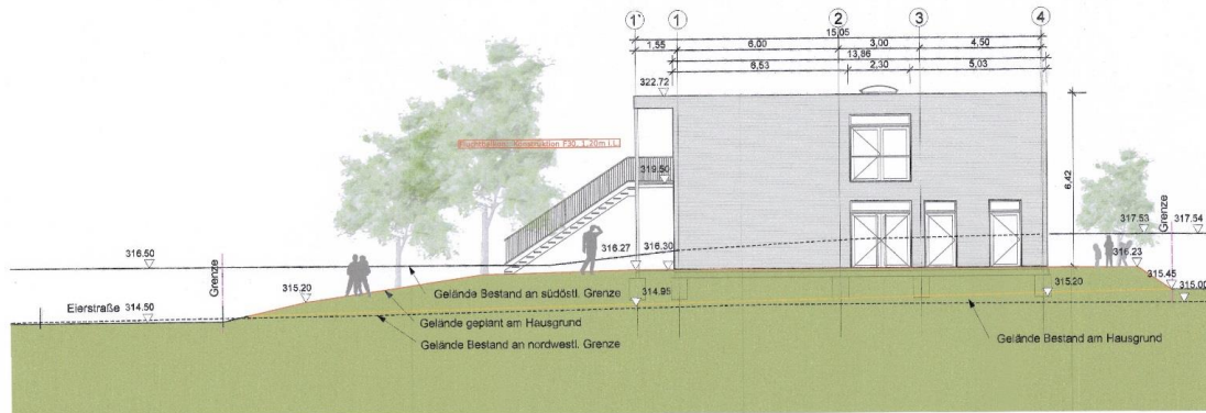
Ansicht Nordwest
