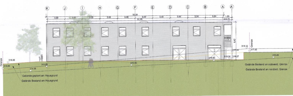
Ansicht Südwest
