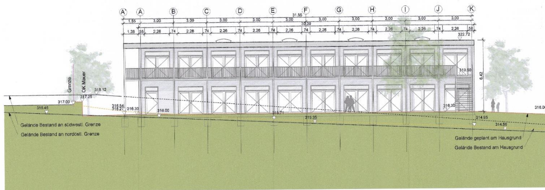
Ansicht Nordost
