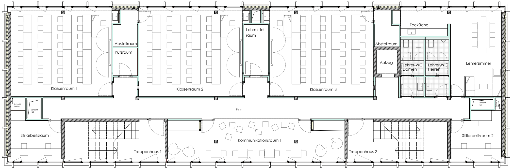
Grundriss 1. Obergeschoss
