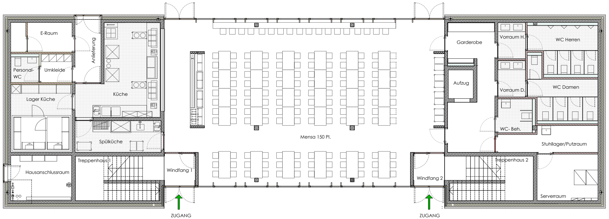
Grundriss Erdgeschoss
