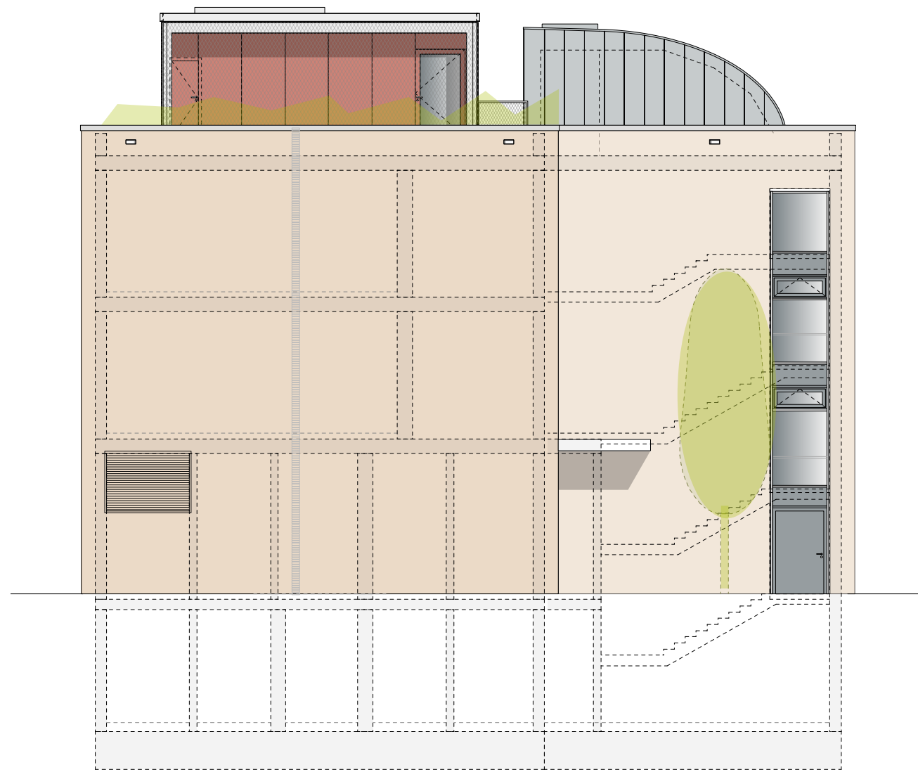
Ansicht Nord
