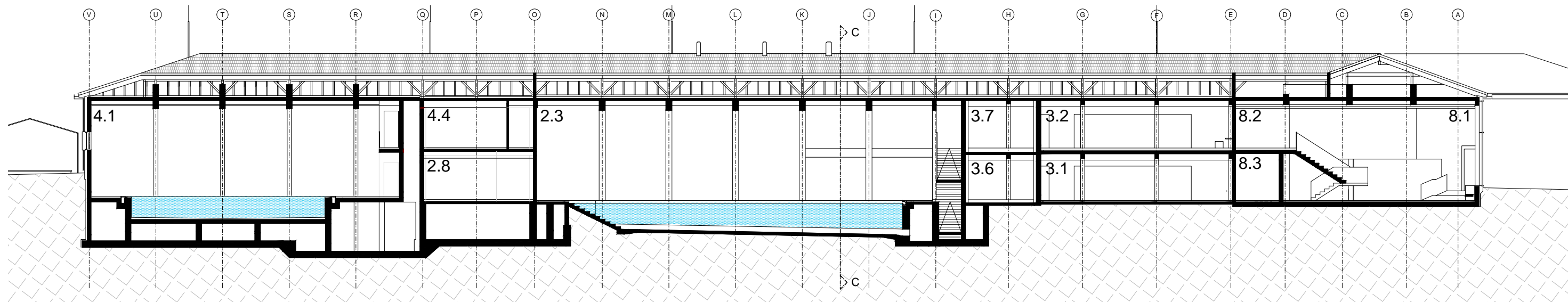
Schnitt 2 - 2
