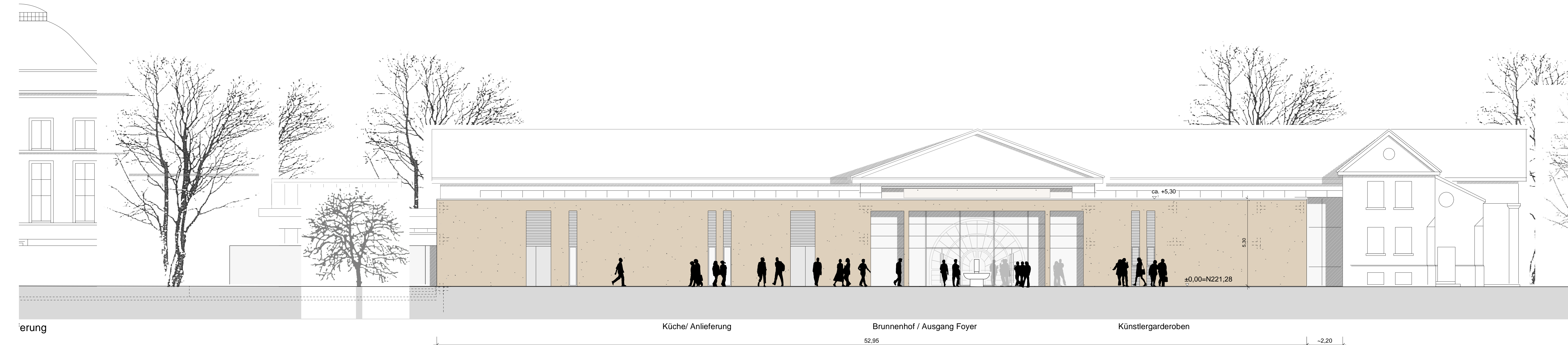
ANSICHT OSTEN
