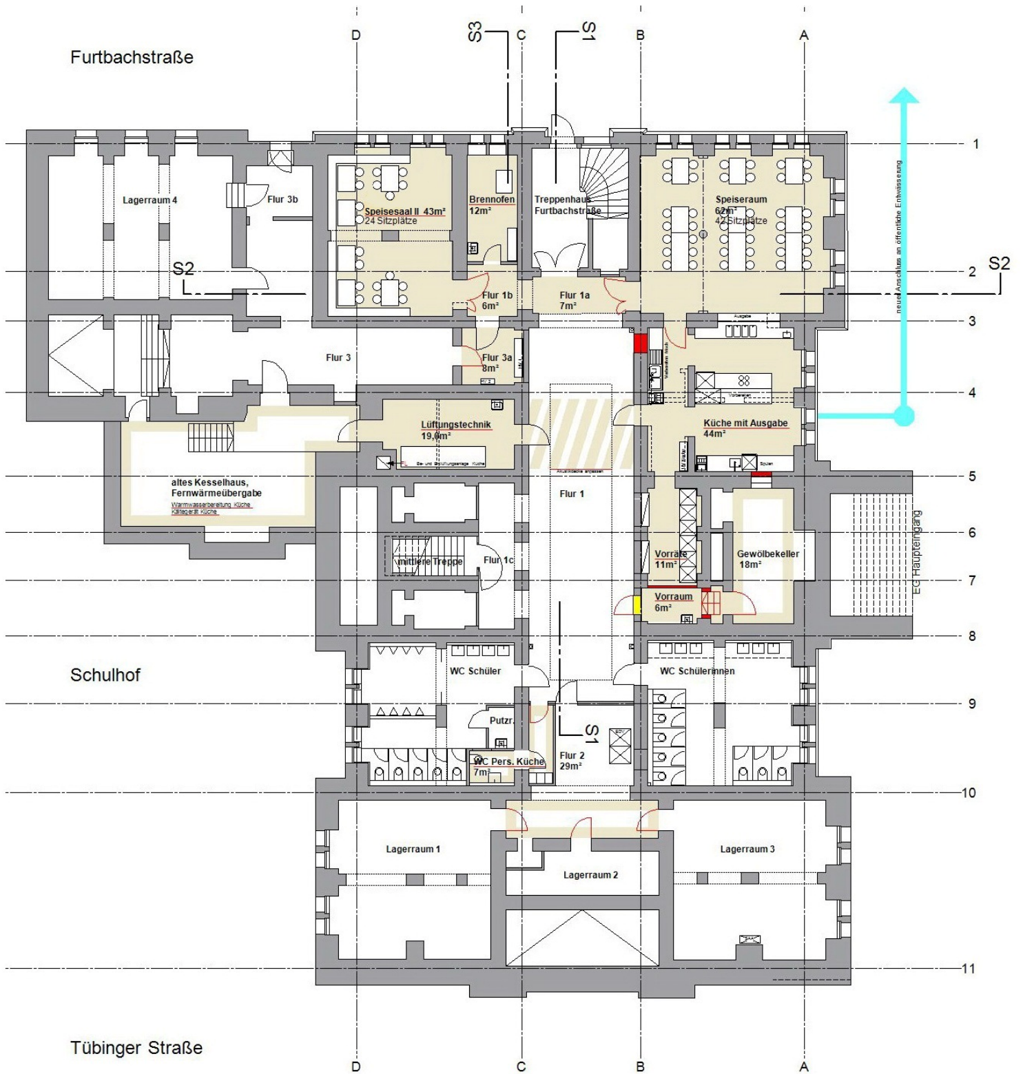
Grundriss Umbau
