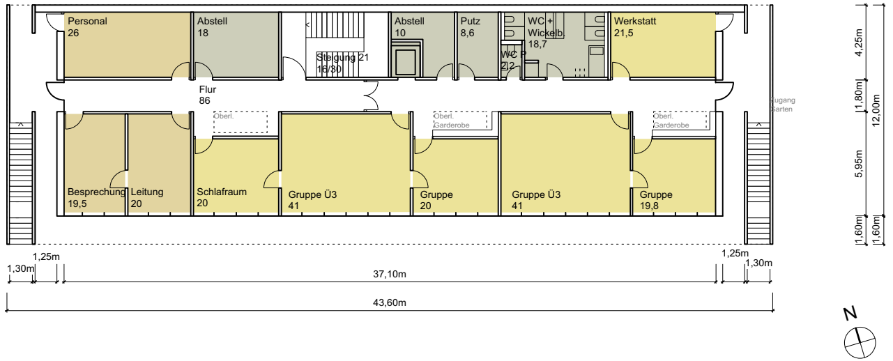
Grundriss Obergeschoss
