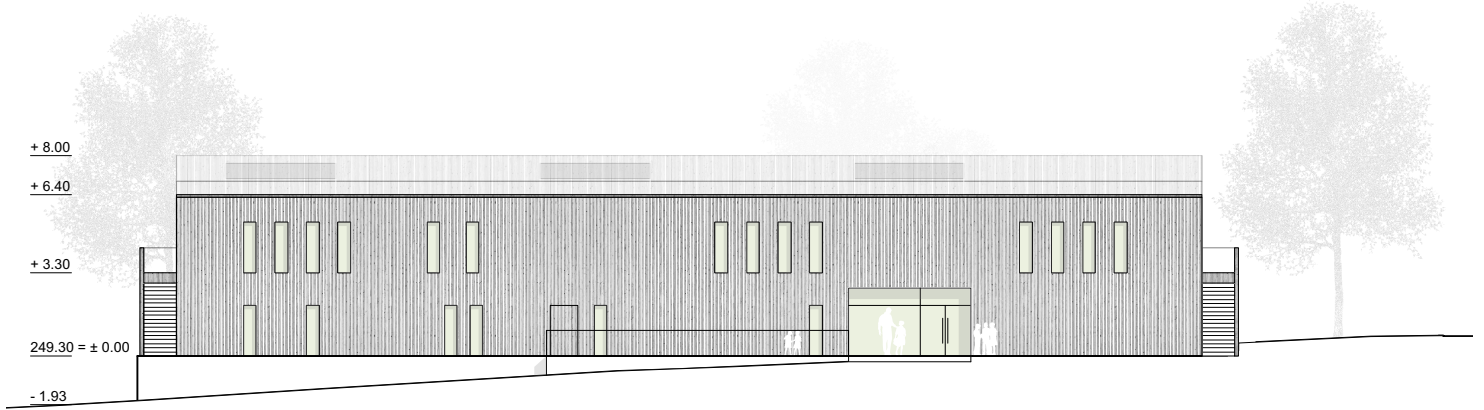
Ansicht Nord
