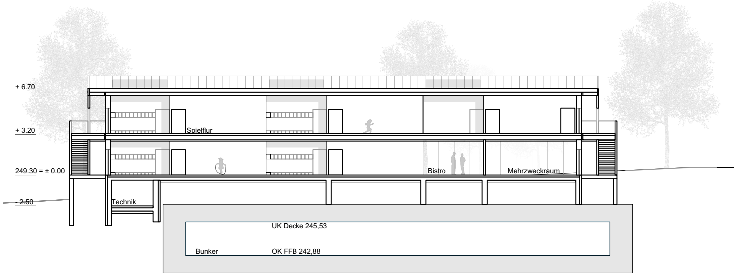
Schnitt BB
