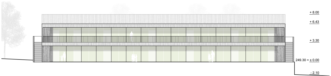
Ansicht Süd
