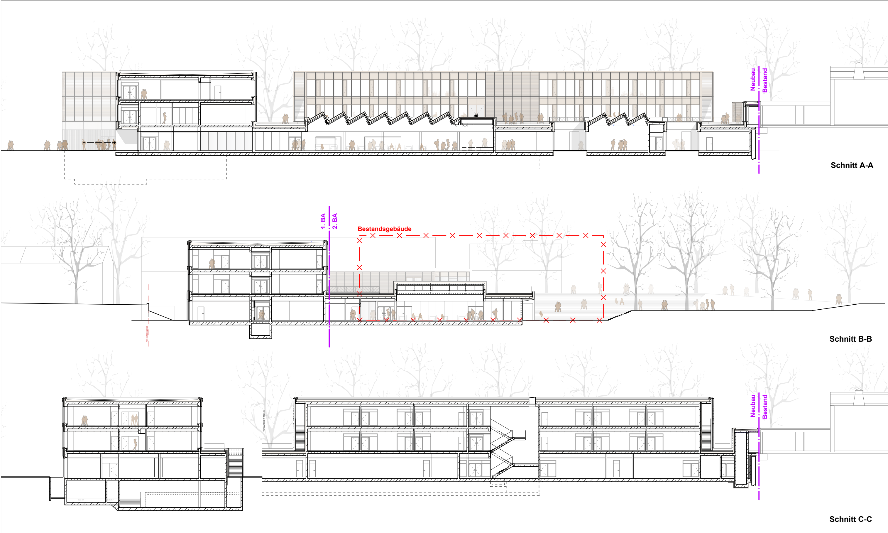
Schnitte
