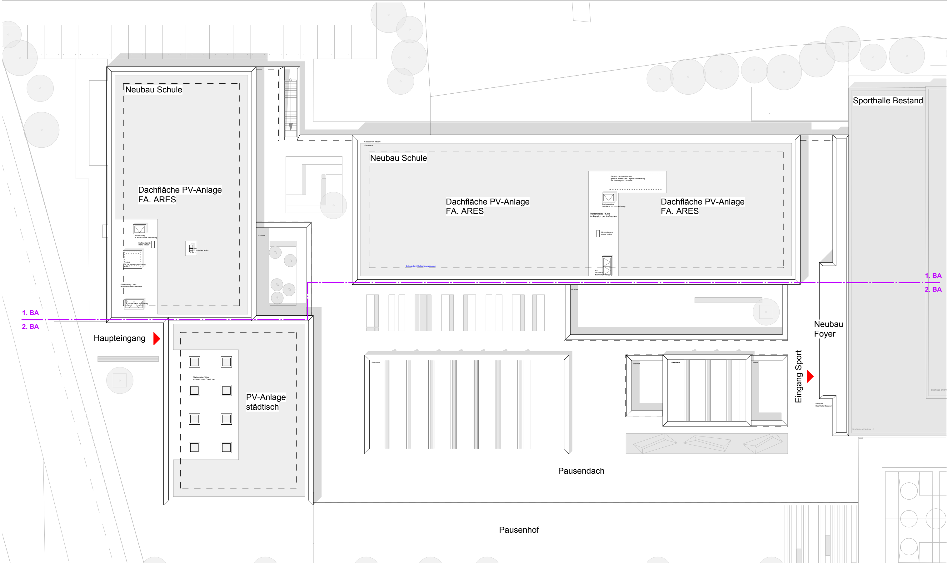
Dachaufsicht
