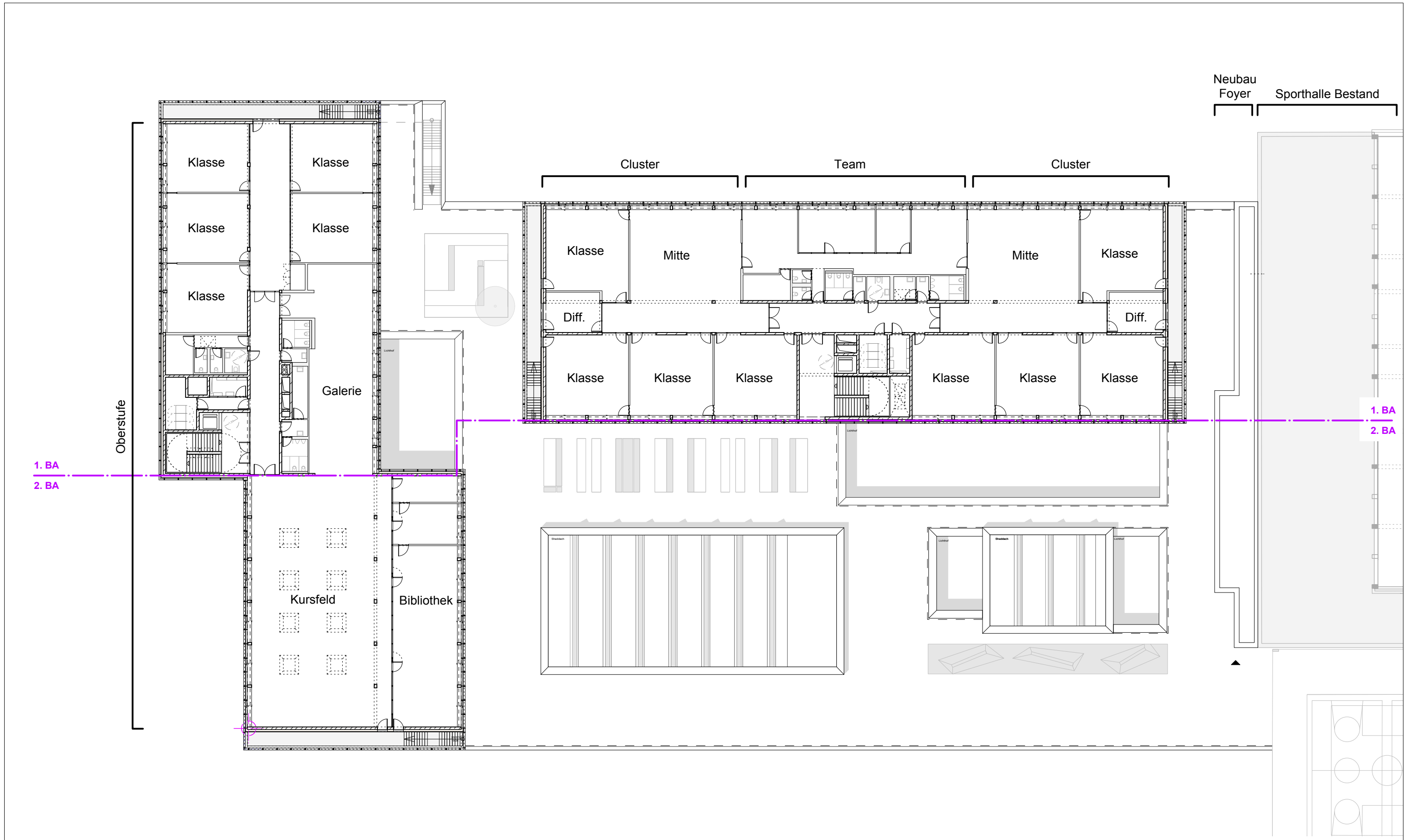
Grundriss 2. Obergeschoss
