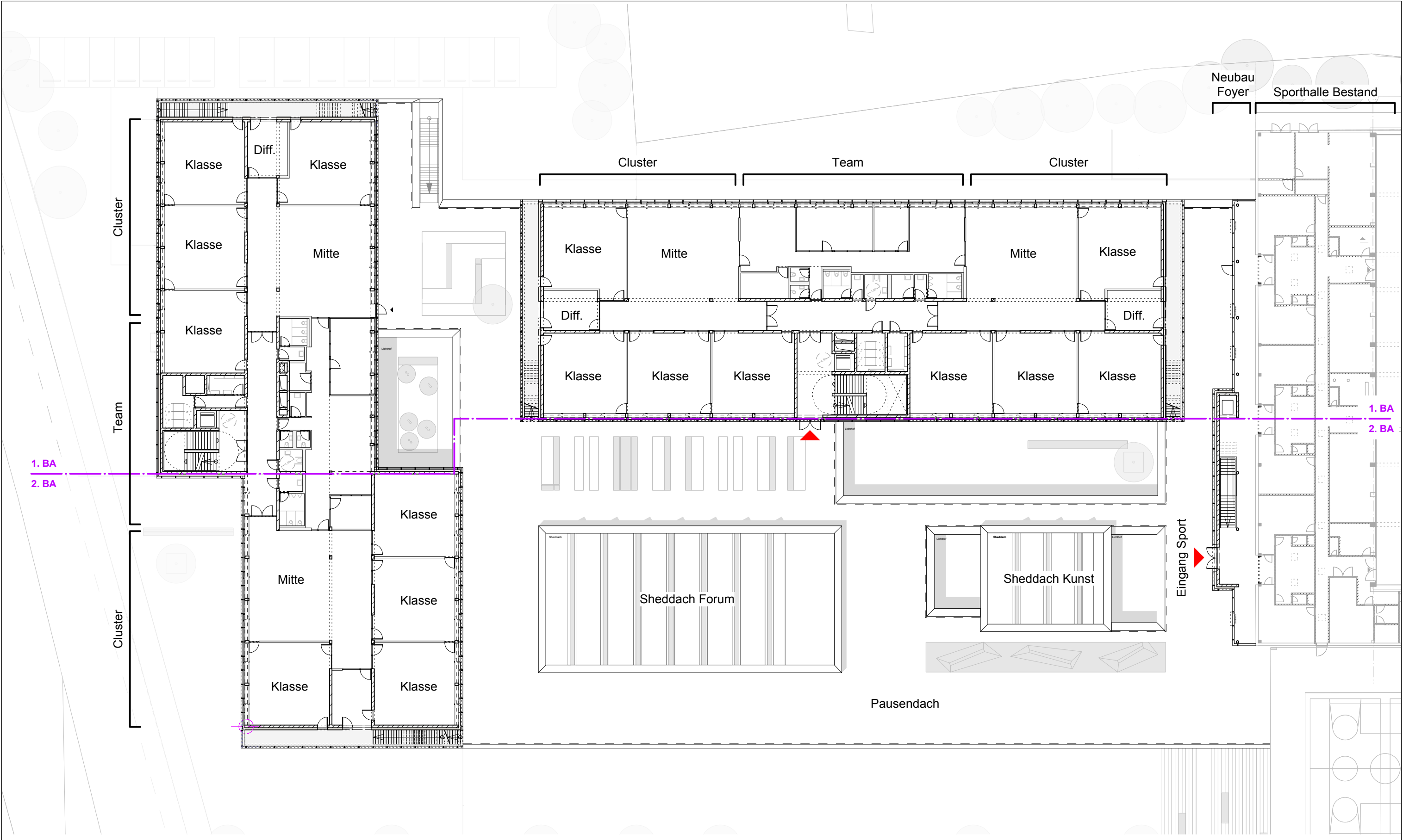
Grundriss 1. Obergeschoss
