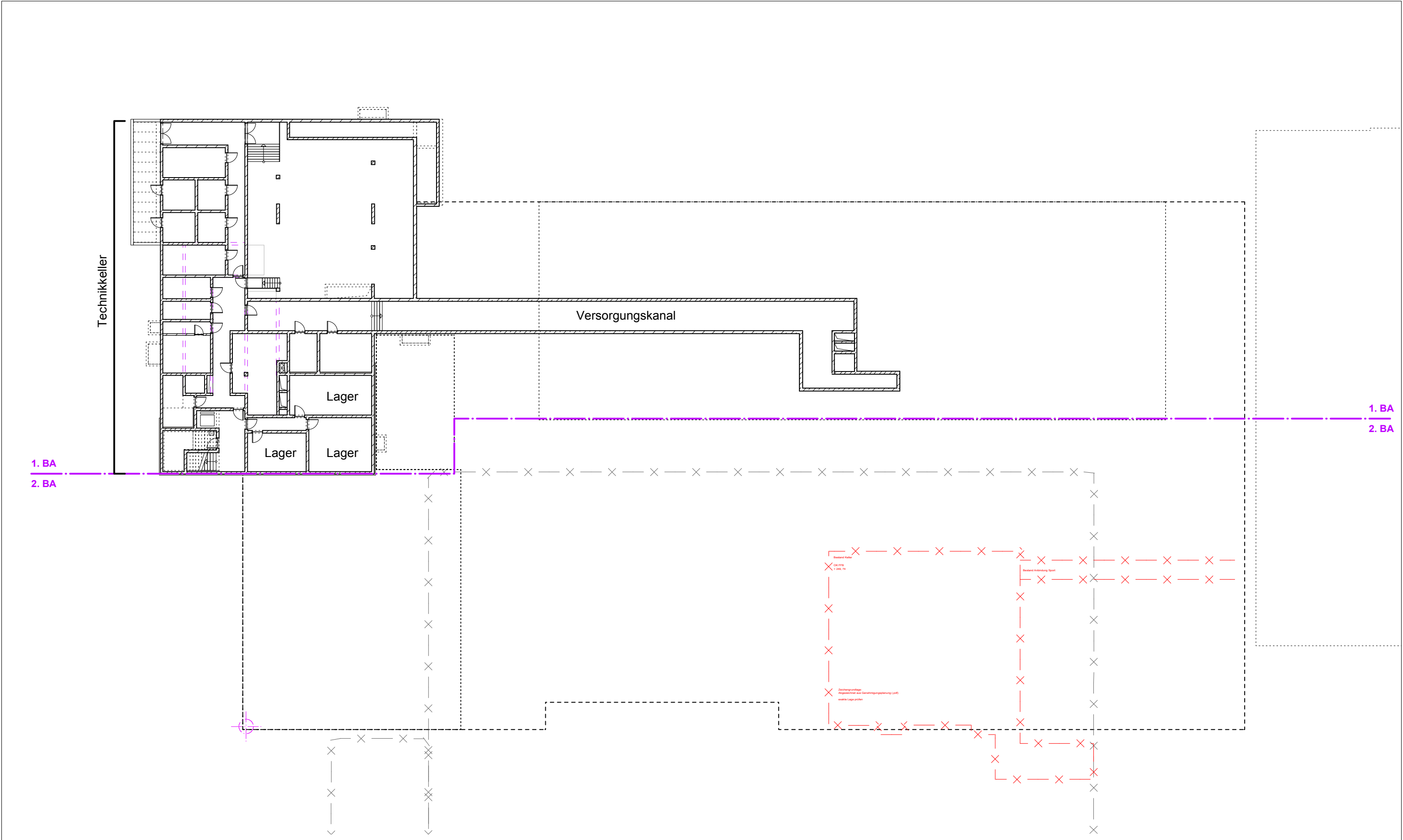
Grundriss Untergeschoss
