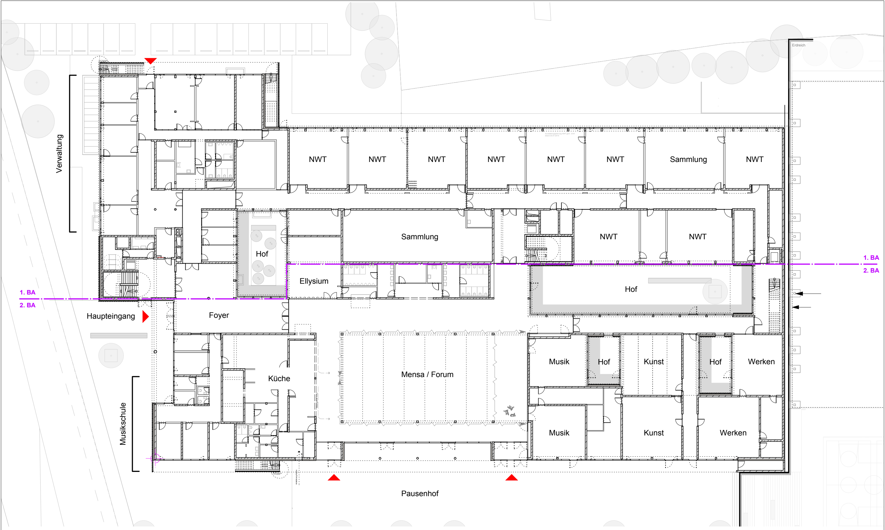
Grundriss Erdgeschoss
