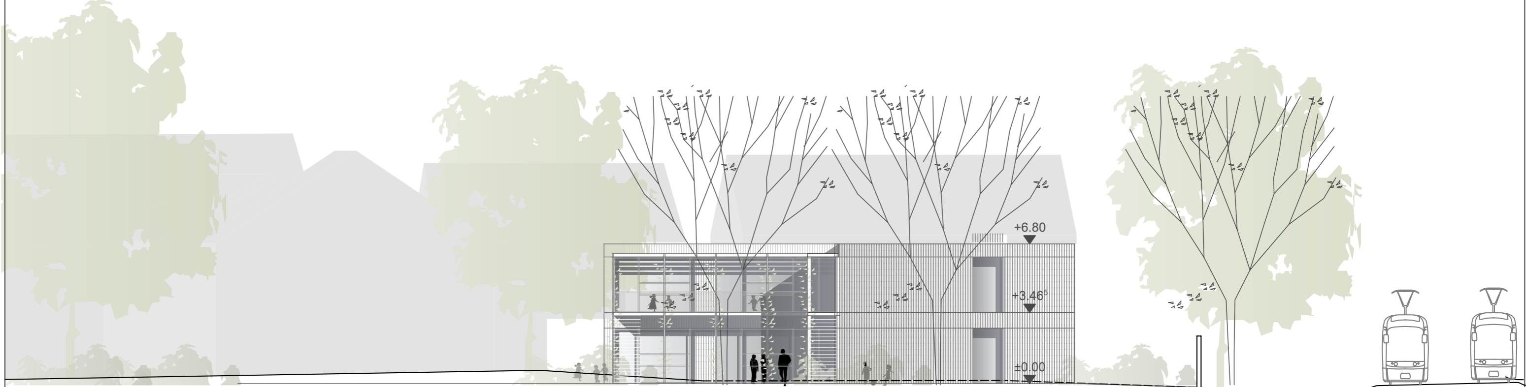
Ansicht Nord-Ost 1:200
