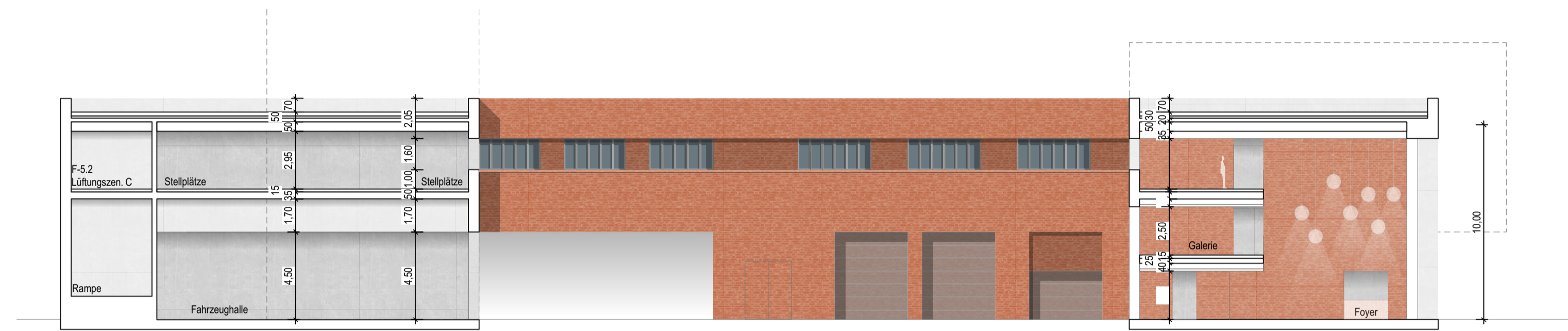
Osten - Bauteil D
