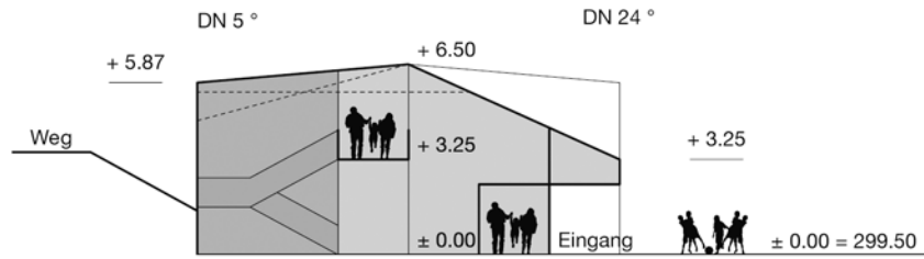
Schnitt B-B 1/200
