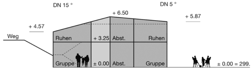
Schnitt C-C 1/200
