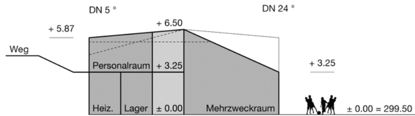
Schnitt A-A 1/200
