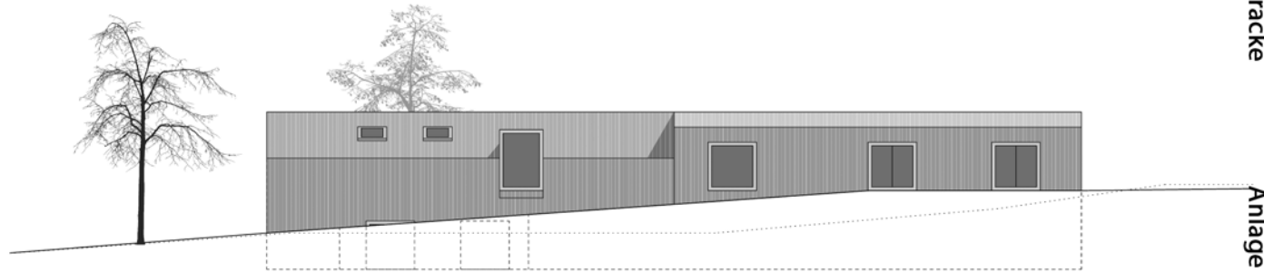
Ansicht Nord 1/200
