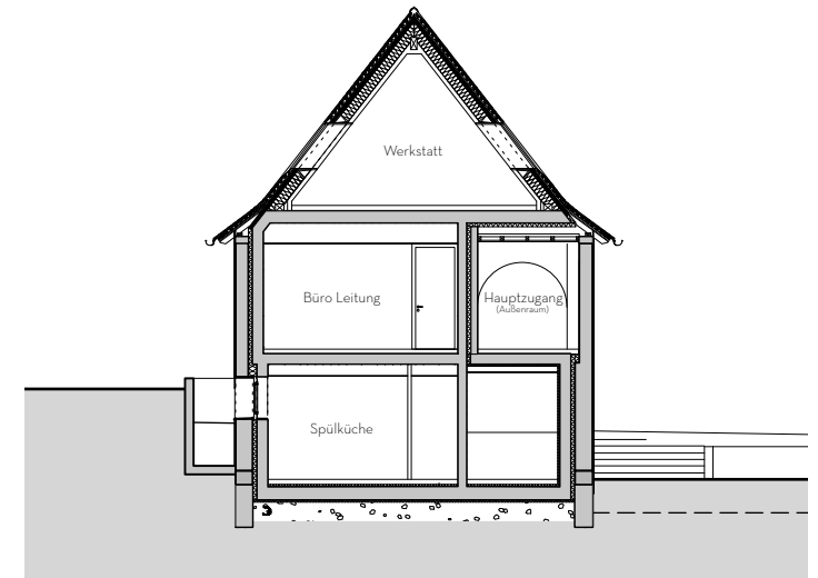
QUERSCHNITTE - M 1:200 GRDRs 900/2016 - Anlage 4.5
