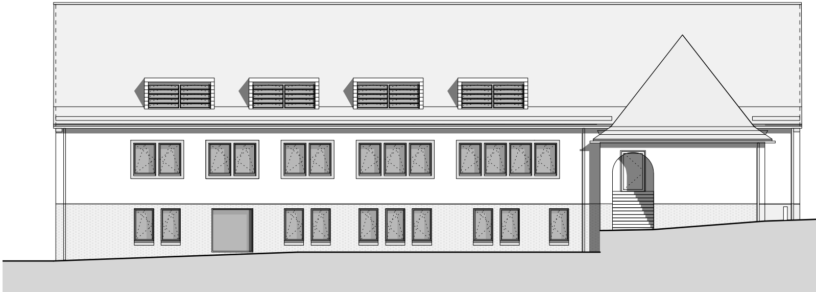
NORDOSTANSICHT
