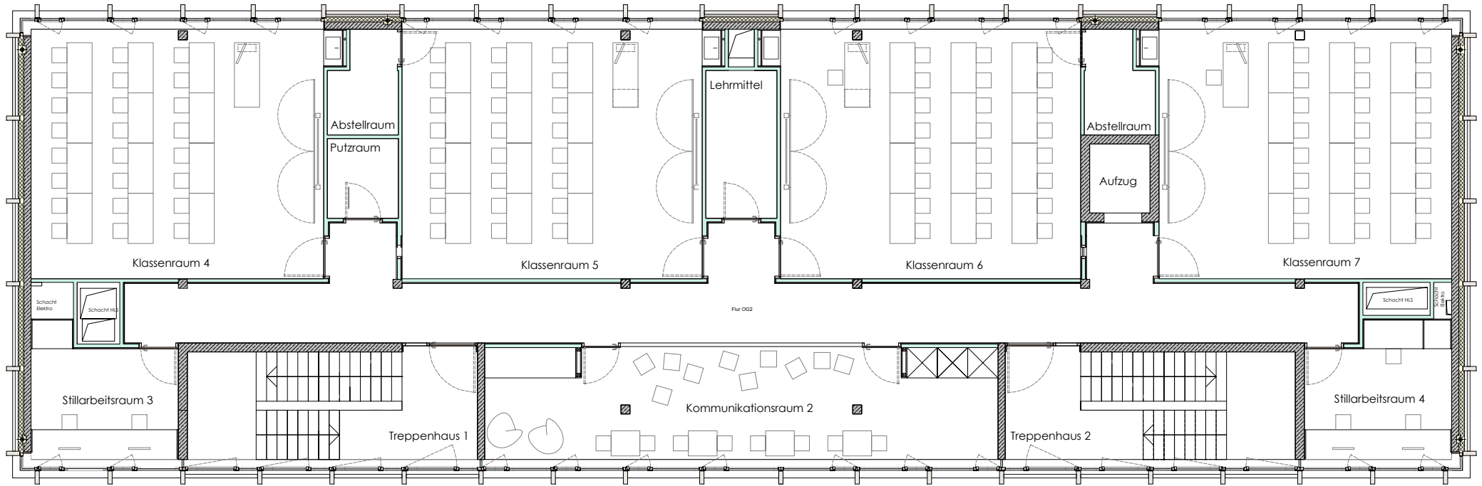
Grundriss 2. Obergeschoss
