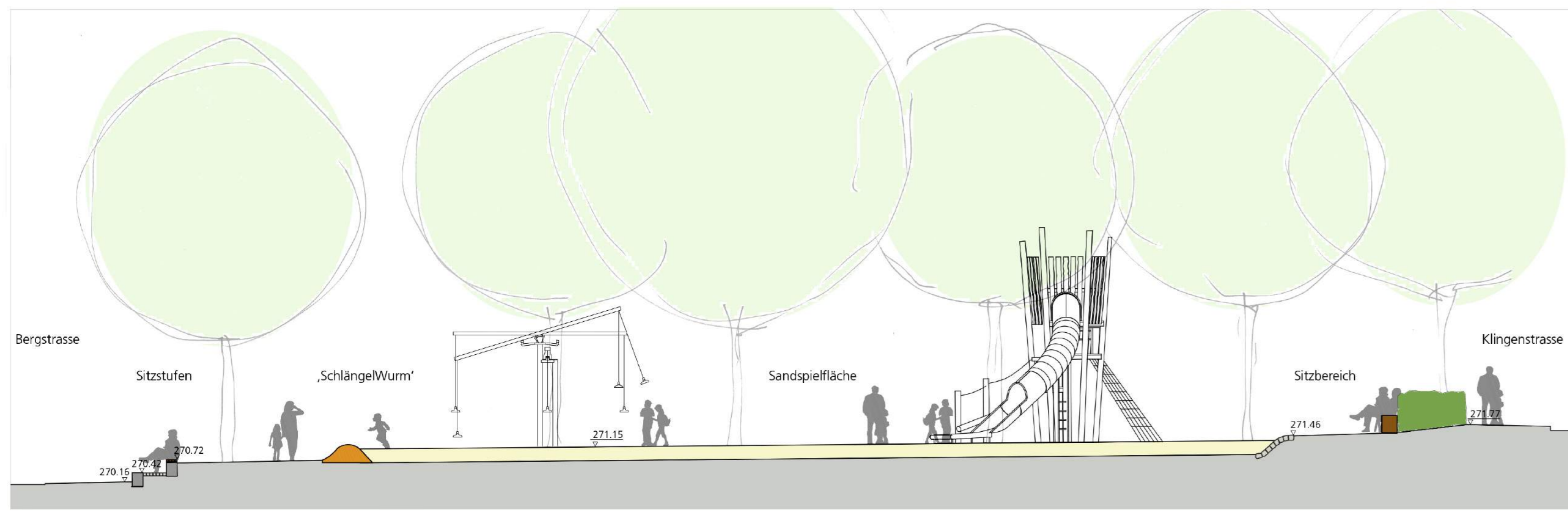
Schnittansicht 1-1 M 1:100
