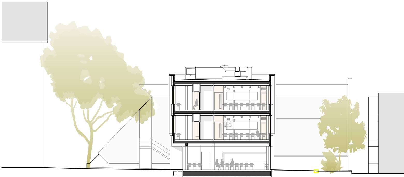
D'Inka Scheible Hoffmann Architekten BDA - Entwurf Mensa und Erweiterung Zeppelin-Gymnasium, Stuttgart Ost - Ansicht Süd-Ost und Querschnitt
