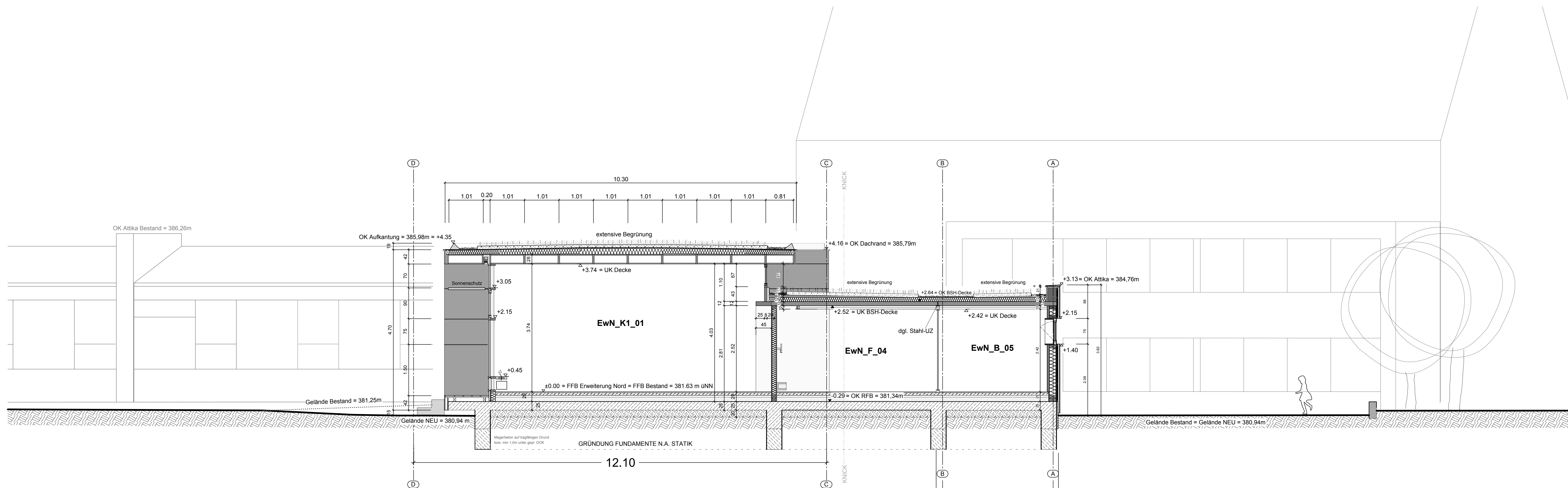
SCHNITT 2-2
