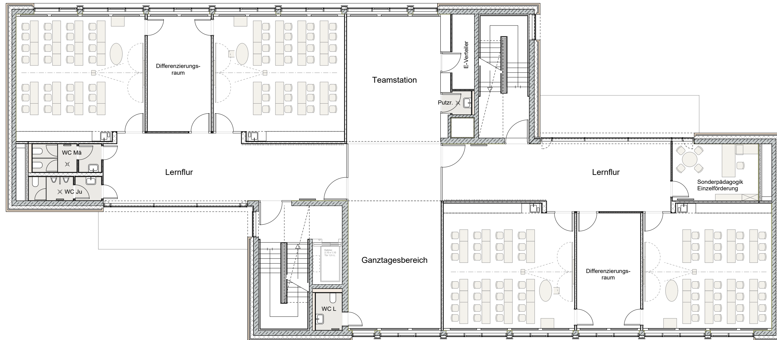
Grundriss 2. Obergeschoss
