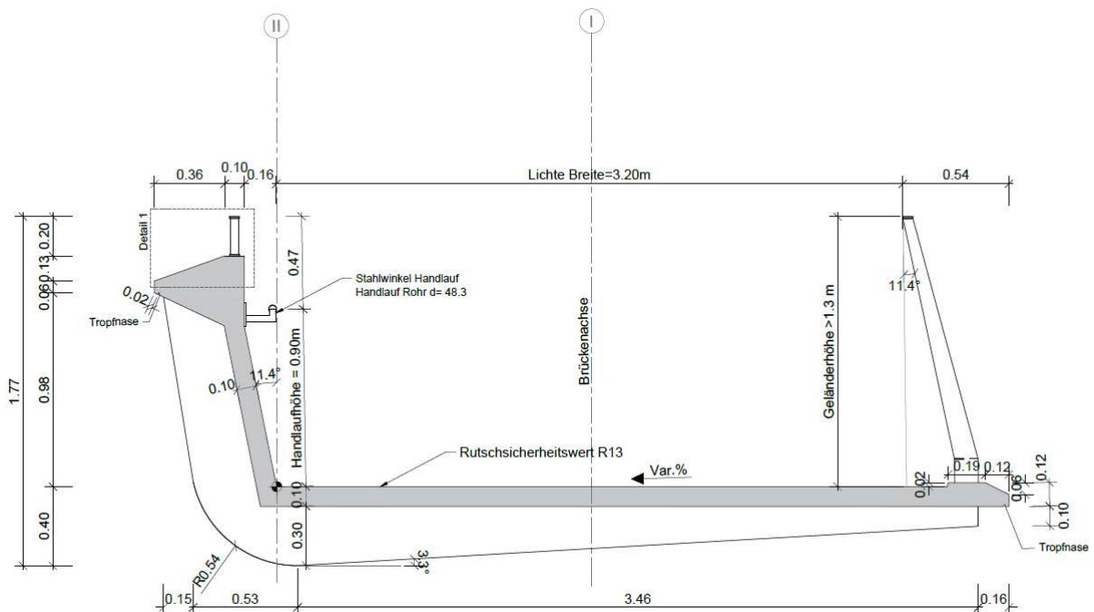
Abb.2: Querschnitt der geplanten Geh- und Radwegbrücke über die Ludwigsburger Straße
