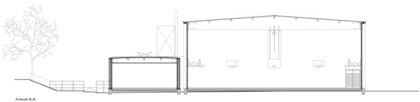
Querschnitt
